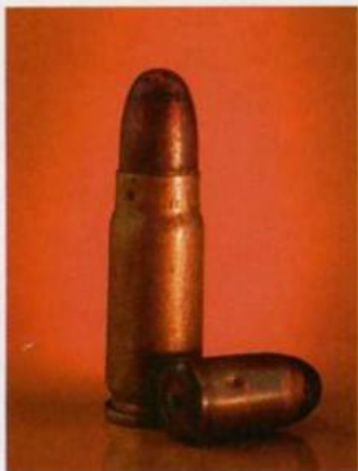
7,62-мм патрон образца 1930 года с броневойно- зажигательной пулей П-41. Гильза — латунная
