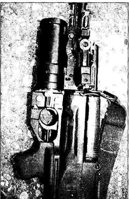
Подствольный гранатомет ПП-25 «Костер»
