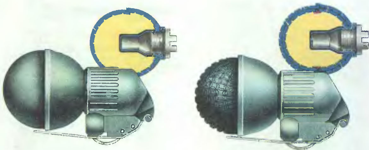
Ручные осколочные гранаты — оборонительная РГО и наступательная РГД (СССР)
