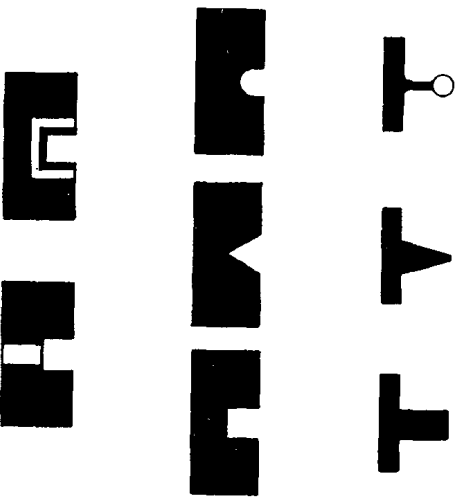
Формы мушек и цетиков открытых прицельных механических приспособлений. В нижнем ряду — цетики со светящимися жемчугами для стрельбы в сумерки или в темных помещениях
