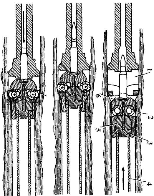
Работа системы автоматики и затвора канала ствола пулемета МГ 43 (МГЗ): 1 — ствольная муфта, 2 — запирающие ролики, 3 — боевая личинка затвора, 4 — остои затвора, 5 — муфта ударника, 6 — зеркала затвора, 7 — отпирывающие кулачки
