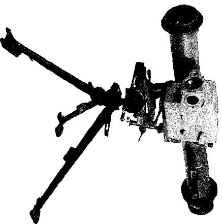
Универсальная установка РПЛ-27
