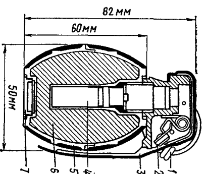
Разрез ручной гранаты RVB NR446 (Бельгия): 1 — предохранительная чека с колышком, 2 — курок, 3 — предохранительный рычаг, 4 — детонатор, 5 — пластиковый корпус с ребрами жесткости, 6 — разрывной заряд, 7 — пробка
