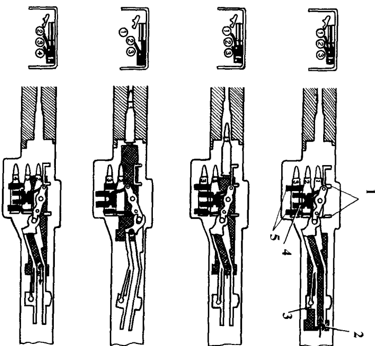
Работа системы питания пулемета МАГ: 1 — направляющие прижимника, 2 — ролик затвора, 3 — крышка, 4 — лента, 5 — внутренние пальцы
