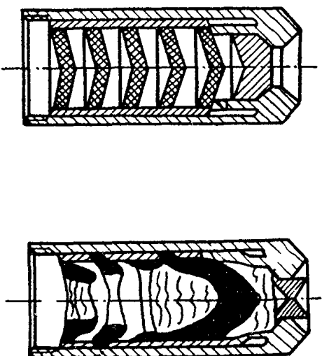
«Пулеуправляватель» после выстрела. Пуля осаживается носовой перегородкой
