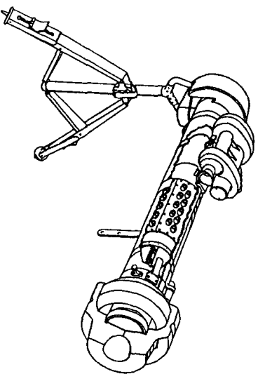
Схема устройства ТПК «Драгон»
