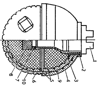
Оборонительная ручная граната РГО: 1 — пробка, 2 — манжета, 3 — опатка, 4 — полусфера, 5 — разрывной заряд, 6 — полусфера, 7 — прокладка, 8 — демонстрационная шашка, 9, 10 — внутреннее полусфера
