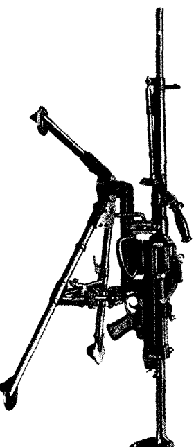
Единый пулемет ААТ
