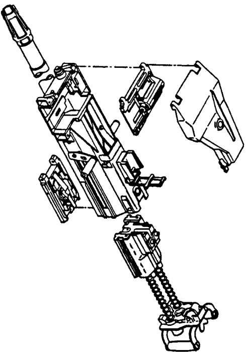
Неполная разборка гранатомета Mk19
