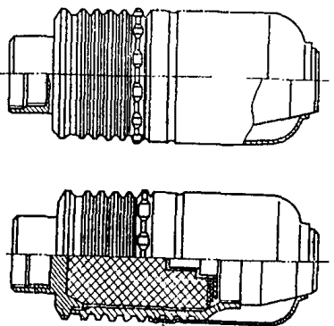
Схема устройства выстрела ВОГ-25
