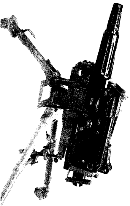
Автоматический гранатомет LAG-40 «Санта-Барбара»
