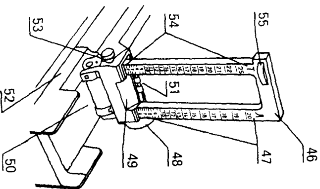
Ручной прицел пулемета: 46 — прицельная планка, 47 — шкала для легкой пули, 48 — маховичок ходового винта, 49 — хомут, 50 — пружина рамки, 51 — цетик, 52 — основание прицела, 53 — цетика, 54 — шкала для тяжелой пули, 55 — маховичок винта точной установки
