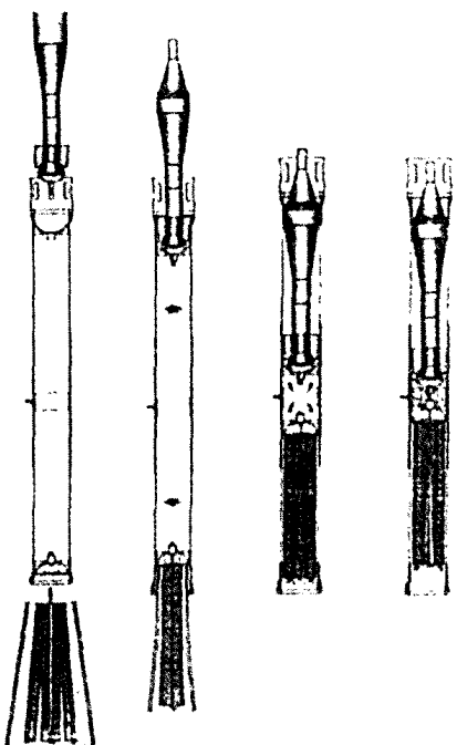
Принцип метания гранаты РПГ «Армбруст»
