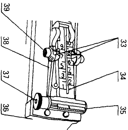
Секторный прицел (ручной прицел РПК): 33 — хомут, 34 — прицельная планка, 35 — цетик, 36 — предохранитель цетика, 37 — маховичок винта цетика, 38 — прицельная колодка, 39 — цетика
