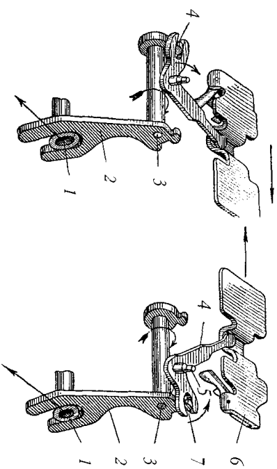
Схема работы подающего механизма пулемета ДШКМ при правой подаче ленты (справа): слева — работа механизма при левой подаче ленты. 1 — рукоятка затворной рамы, 2 — рычаг затворной рамы, 3 — ось рычага рамы, 4 — рычаг ползунка, 5 — ось рычага ползунка, 6 — ползун, 7 — выступ рычага рамы
