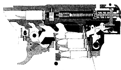
Схема ударно-спускового механизма Р99
