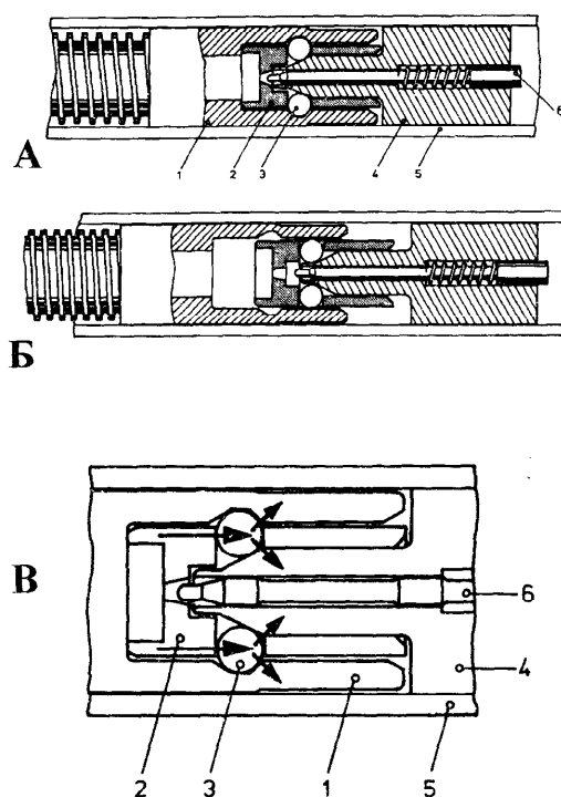
Схема работы автоматики с полусвободным затвором пистолета Р9НК (ФРГ): 1 — ствол, 2 — боевая личинка затвора, 3 — шарики, 4 — остов затвора, 5 — кожух затвора, 6 — ударник А — перед выстрелом; Б — процесс отпирания; В — расклад сил при отпирании канала ствола.
