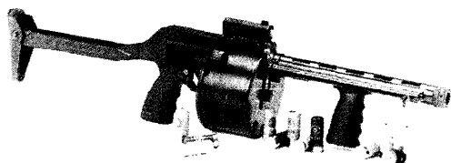
Боевое гладкоствольное револьверное оружие «Протекта»
