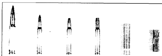
Различные варианты штатных и опытных патронов: 7,62-мм М80; 5,56-мм патроны, использовавшиеся в программе ACR, — М855; двухпульный «Калт Дуплекс» в гильзе штатного 5,56х45; патрон АМ со стреловидной подкалиберной пулей в гильзе штатного 5,56х45; телескопический патрон «Штейр-Манлихер» со стреловидной подкалиберной пулей в пластиковой гильзе; безгильзовый патрон «Динамит-Нобель»
