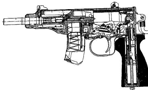
Разрез малого пистолета-пулемета M84 «Застава» (копия «Скорпиона»)
