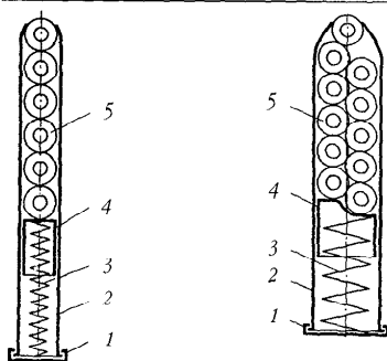
Схема двухрядного магазина (шахматное расположение патронов): 1 — крышка, 2 — корпус, 3 — пружина подавателя, 4 — подаватель, 5 — патрон
