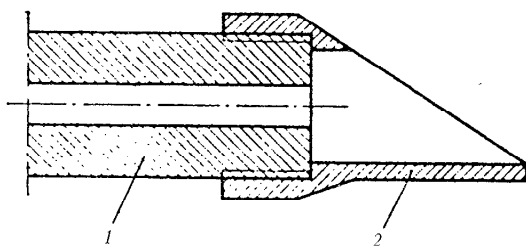
Надульник-компенсатор: 1 — ствол, 2 — компенсатор активного действия
