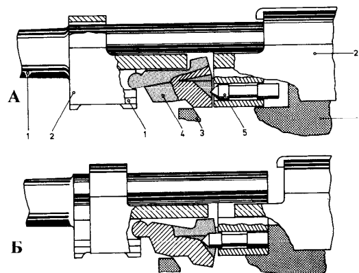
Схема работы системы затвора пистолета Р38 (Р1) «Вальтер»: А — канал ствола заперт, Б — канал ствола открыт; 1 — ствол, 2 — затвор, 3 — рамка, 4 — личинка, 5 — отпирающий стержень
