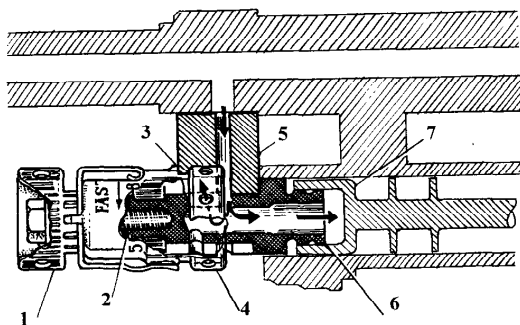
Газовый регулятор пулемета MAG (Бельгия): 1 — регулировочная втулка, 2 — винт подачи, 3 — обойма, 4 — выпускное кольцо, 5 — входной патрубок, 6 — газовая муфта, 7 — газовый поршень
