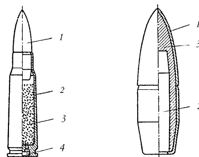
Устройство промежуточного патрона (автоматного) обр. 1943 г.: 1 — пуля, 2 — гильза, 3 — пороховой заряд, 4 — капсюль
