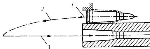
Схема подачи патрона из ленты с замкнутым звеном: 1 — извлечение патрона из ленты, 2 — снижение патрона на линию досылания, 3 — досылание патрона
