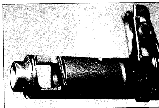
Пламегаситель-компенсатор АК-74
