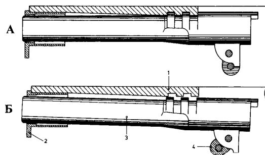
Работа автоматики и системы запирания пистолета M1911A «Кольт»: А — ствол заперт, Б — отпирание; 1 — затвор-кожух; 2 — отулка ствола, 3 — ствол, 4 — серьга ствола
