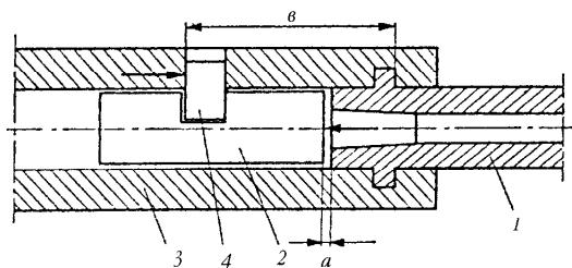
Затирание канала ствола с помощью клина: 1 — ствол, 2 — затвор, 3 — ствольная коробка, 4 — поперечно движущийся клин, а — зазор между пеньком ствола и зеркалом затвора, в — длина узла затирания
