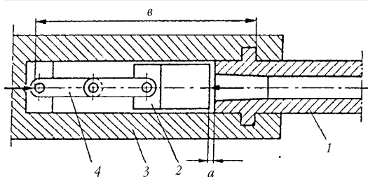
Затирание канала ствола шарнирно-рычажной системой: 1 — ствол, 2 — затвор, 3 — ствольная коробка, 4 — система рычагов, а — зазор между пеньком ствола и зеркалом затвора, в — длина узла затирания
