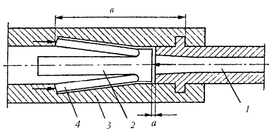
Затирание канала ствола разведением боевых упоров затвора: 1 — ствол, 2 — затвор, 3 — ствольная коробка, 4 — качающийся боевой упор, а — зазор между пеньком ствола и зеркалом затвора, в — длина узла затирания
