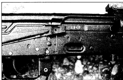
Переводчик-предохранитель АК-74 в положении «ПР»
