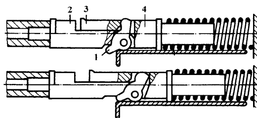
Схема работы рычажного ускорителя: 1 — качающийся рычаг, 2 — ствол, 3 — боевая личинка затвора, 4 — оков затвора
