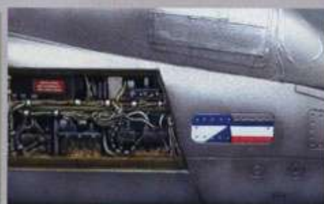
▲右側の国籍マークは日差しによる温色を表現するため、クリアテックスのクリアホワイトをデカールに直接軽くエアブラシした。ただし四角いカバーの部分のみは新しいままにしてある。
