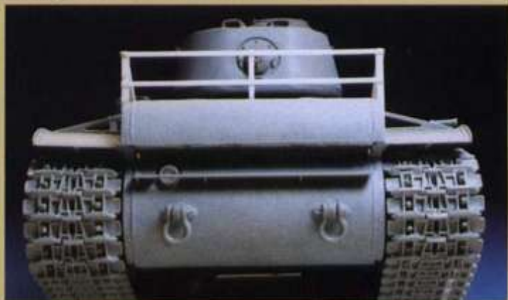
▼キットには車体後部のラックのパーツが入っていないので、プラバンで自作。機関室と車体後部の吸排気口のメッシュはアベールのエッチングパーツに交換した。
