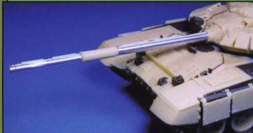
▼ミニアームの砲塔パーツ「T-72BM Turret m1989」には、アルミ製の砲身とレジン製の砲塔本体、リアクティブアーマー、ハッチ、スモークディスチャージャーをセット。
