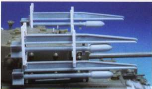
◀▶ RP-3 ロケット弾本 体とランチャーレール は、タミヤ1/48 ソード フィッシュのパーツを、 弾頭部分はエアフィッ クス1/48のスピットファイ ア Mk.22のパーツを使っ た。
