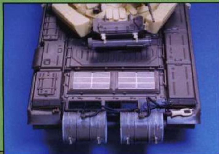
▼エンジンのメッシュと予備燃料タンクの配管類はタミヤのキットに付属している。車体後部のワイヤーロープはカラヤの「Tow Cables」(品番TCR07)を使用。
