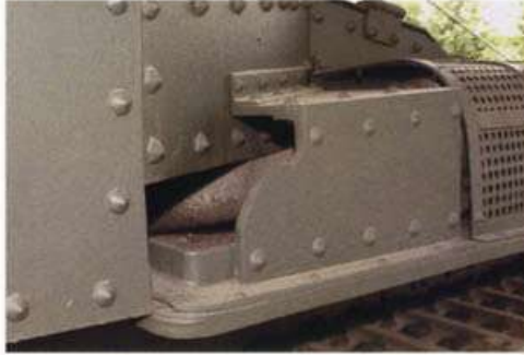
▲マフラー下部のフェンダーには放熱用のスリットが設けられている。▲排気管カバー。写真は車体左側。
