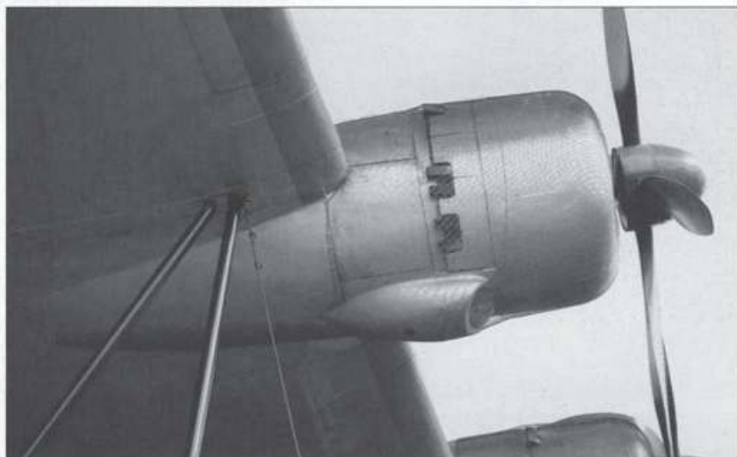
▲右翼外側エンジンカウル。鳥除けのネットが掛けられている。 ▼左翼外側エンジンカウルを下から見上げる。オイルクーラーインテークの形状が良くわかる。
