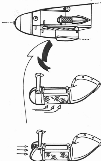
Bf 109 F-2/Trop
