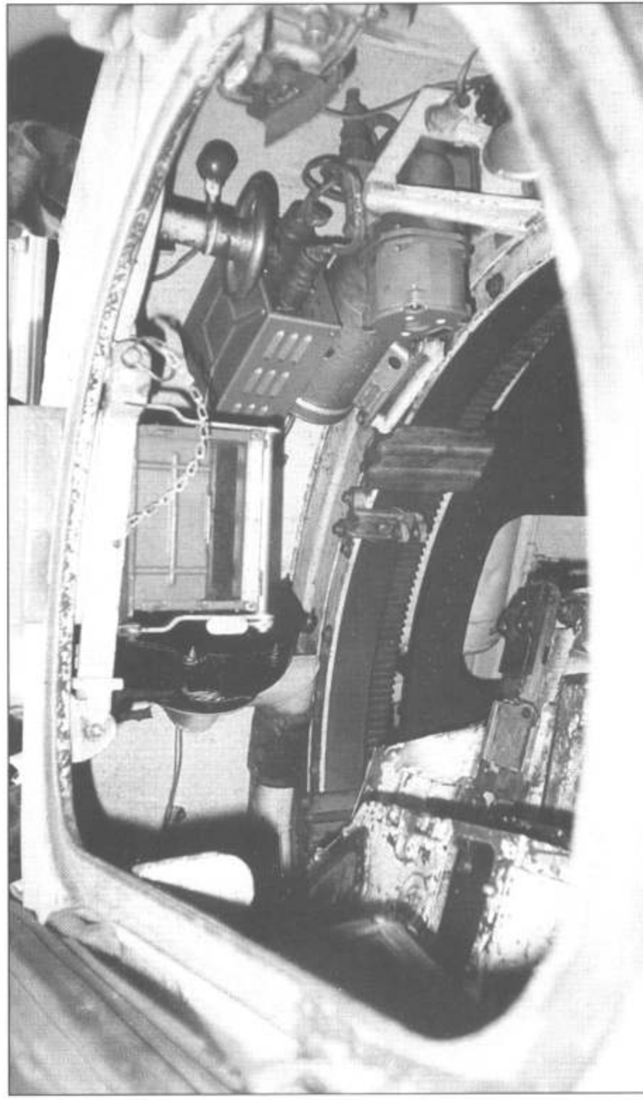
Оборудование на левом борту машины. Спинка левого сидения откинута. Пол окрашен серой краской, борта и крыша корпуса изнутри - белые.
