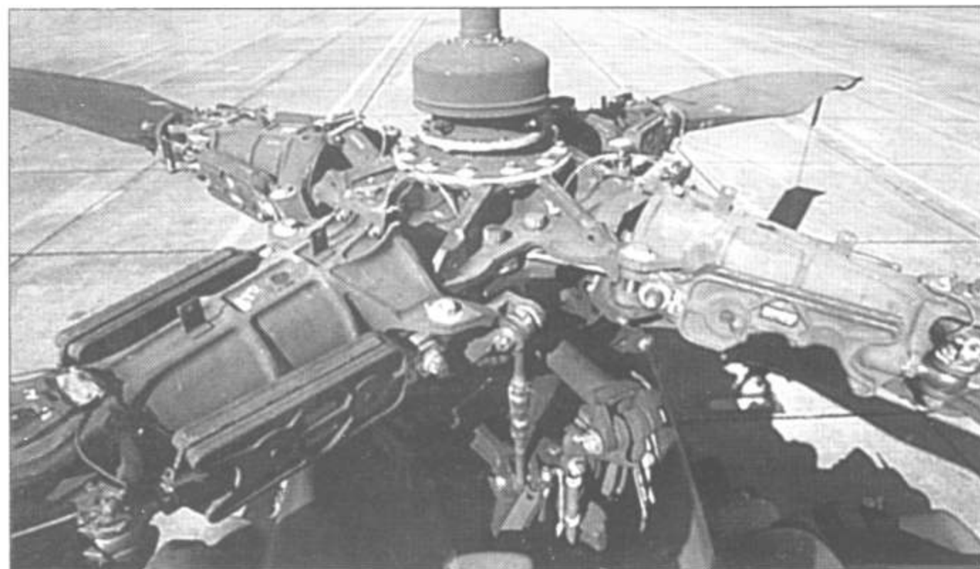
Ротор несущего винта крупным планом
