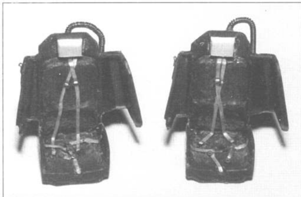
Доработанные кресла пилота и оператора. Подушка заголовника сделана из куска пластика, ремни из фольги, а силовой провод в виде пружины - из тонкой медной проволоки, намотанной на иголку.
