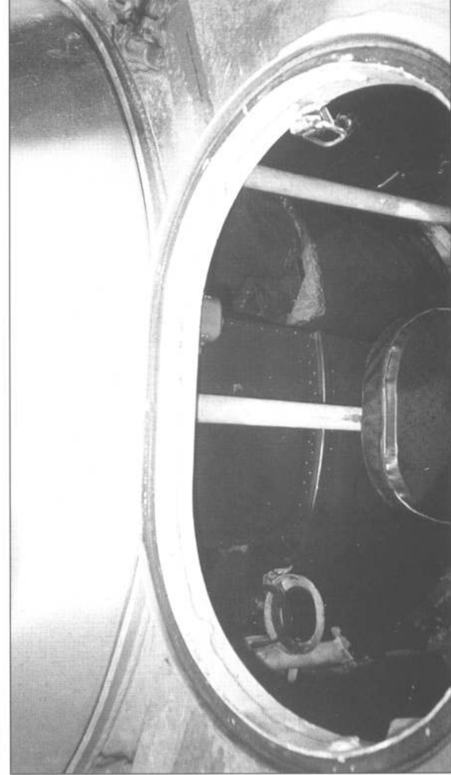
Правый борт. Внутренние элементы гидроннематической подвески закрыты перфорированными кожухами.
