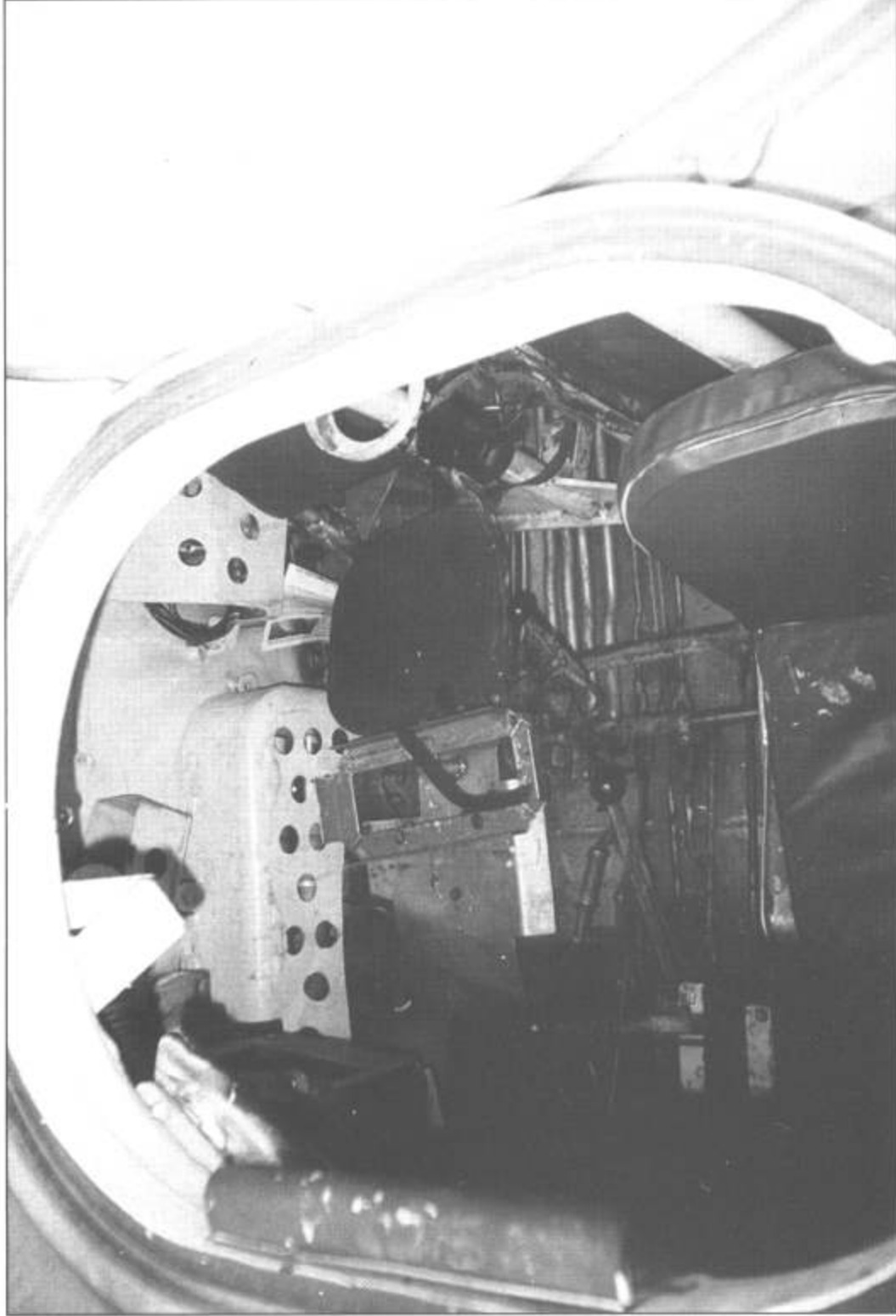
Правый борт. Внутренние элементы гидроннематической подвески закрыты перфорированными кожухами.
