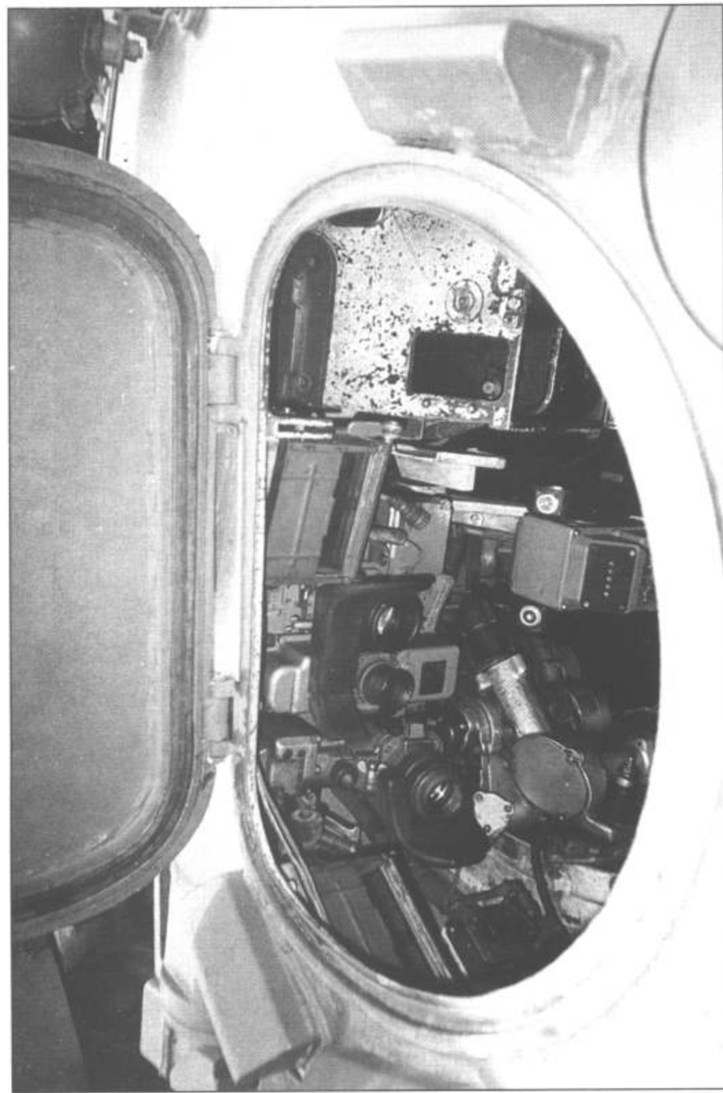
Люк башенного стрелка. Справа - штырь крепления ПУ ПТУР.
