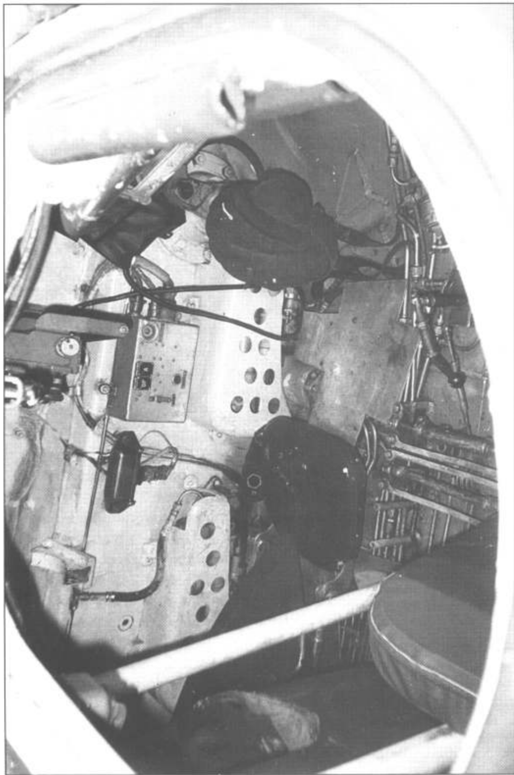
Оборудование на левом борту машины. Спинка левого сидения откинута. Пол окрашен серой краской, борта и крыша корпуса изнутри - белые.
