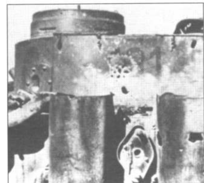
Пример осколочных повреждений легких конструкций танка «Тигр».
