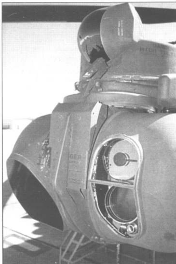
Лазерно-оптическая прицельная система
