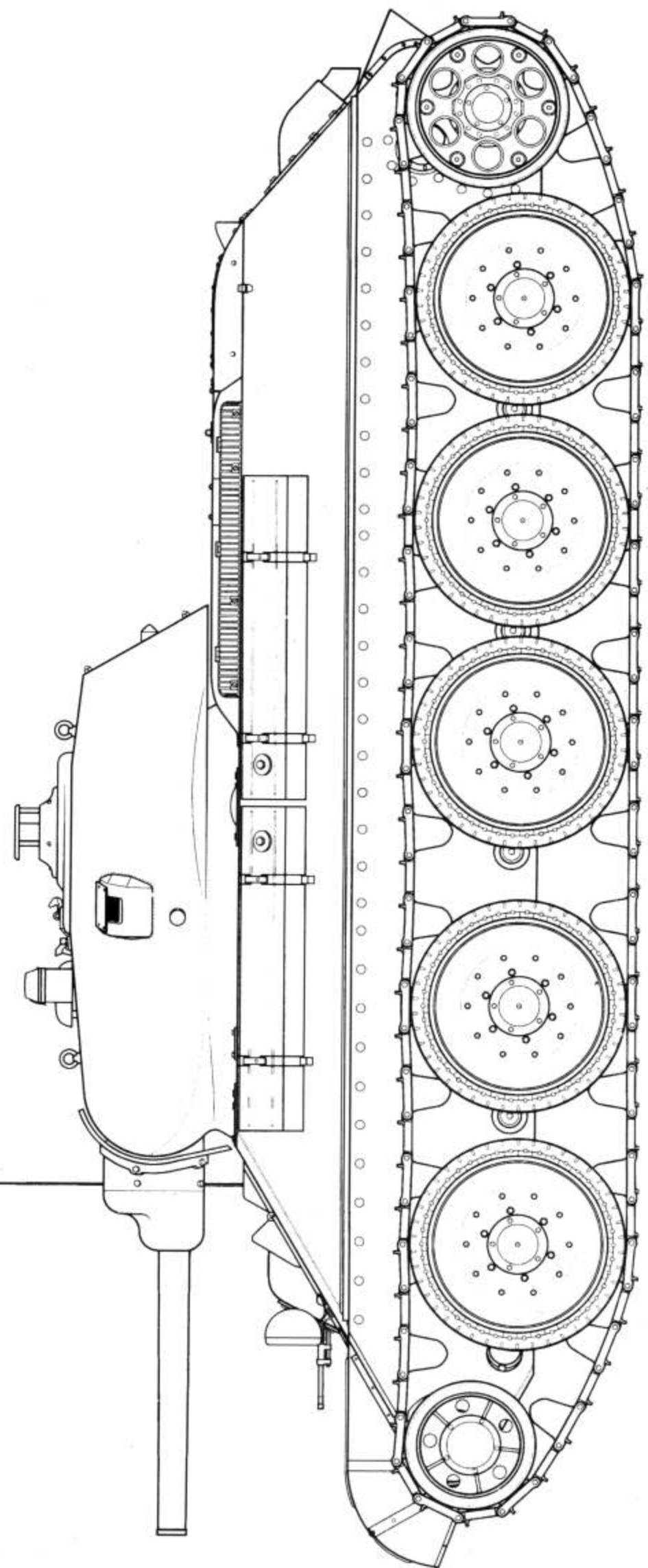
Командирский Т-34 выпуска зимы 1940/41 года. Литая башня с пушкой Л-11.
