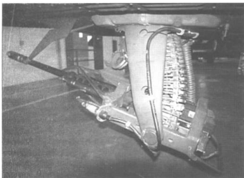
30-мм пушка «Апача» крупным планом
