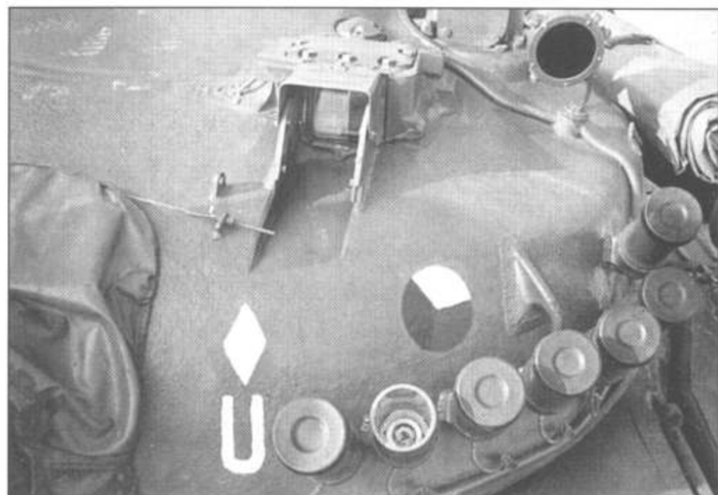
Детали конструкции чешского Т-72М
