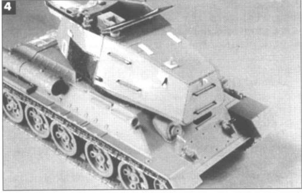
4 Поручни на башне - из набора фирмы Тамия. Обратите внимание на самостоятельно изготовленные петли верхнего люка, антенный ввод и крюки для подъема башни.
