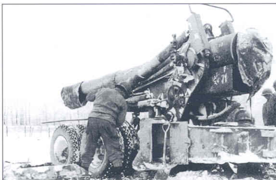
Расчет разворачивает дальнобойное 203-мм орудие М1 на огневой позиции. Положение американских войск в Арденнах в декабре 1944 года было столь незавидным, а погода столь плоха, что для огневой поддержки обороняющихся войск вместо авиации использовалась тяжелая артиллерия (АВЛ).
