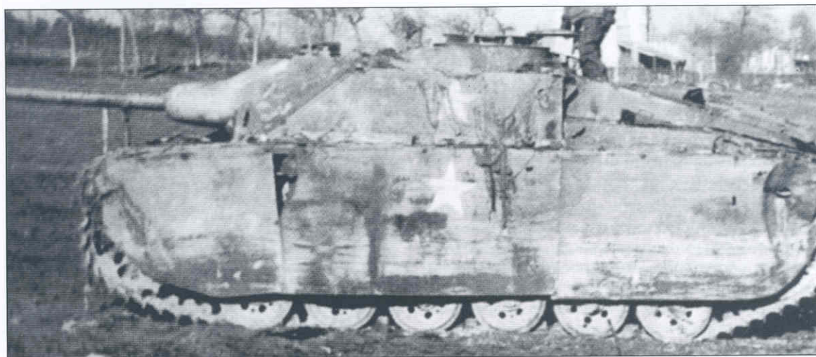
Замаскированные под американскую бронетехнику и брошенные при отступлении германские 75-мм САУ StuG III Ausf. G (с обозначением роты "Ц" 81-го танкового батальона 5-й танковой дивизии) из боевой группы "У" ("игрек") 150-й танковой бригады специального назначения. Район Жеромона, 9-я рота 2150-го батальона, январь 1945 года (АВЛ).
