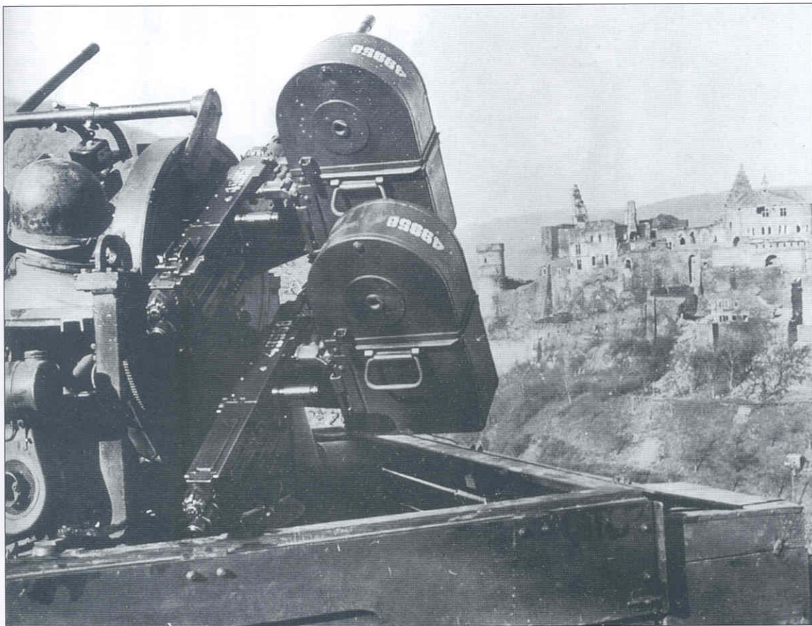
Американская счетверенная зенитная установка М16, состоящая из 4-х крупнокалиберных 12,7-мм пулеметов "Браунинг" на шасси полугусеничного бронетранспортера М3 на боевом дежурстве в небе Люксембурга. Январь 1945 года (АВЛ).
