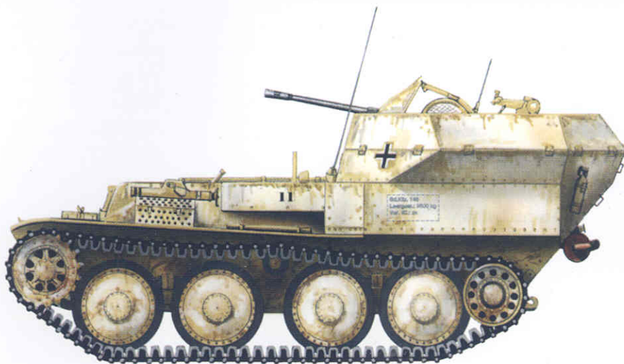
20-мм ЗСУ Flakpanzer Sd.Kfz. 140 неизвестного подразделения из состава 6-й танковой армии СС. 6-я танковая армия СС (в реальности по немецким документам 6-я танковая армия) состояла из 1-го танкового корпуса СС (1 тд СС, 12 тд СС) и 2-го танкового корпуса СС (2 тд СС, 9 тд СС). Арденны, декабрь 1944 года.
