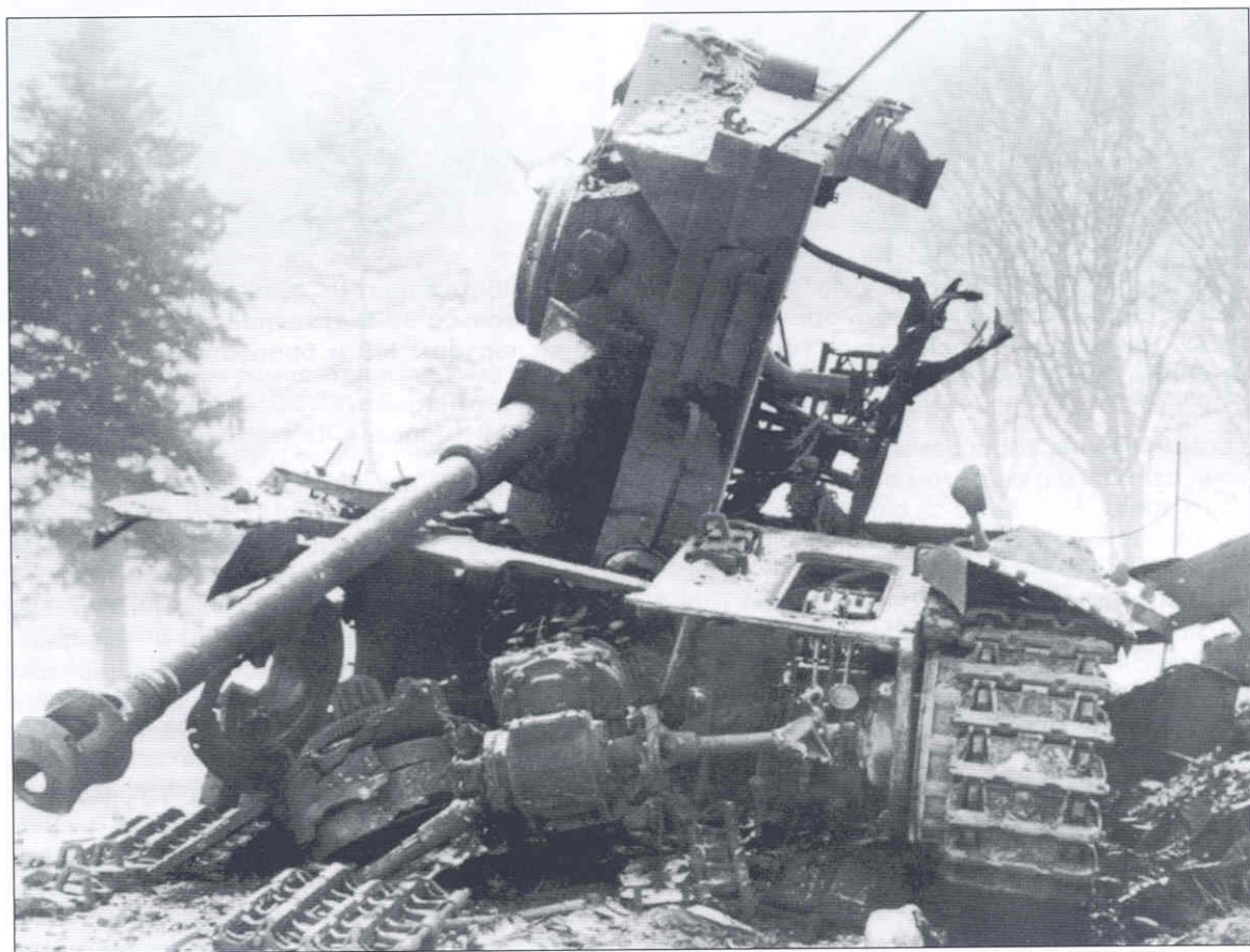
Остатки танка Pz.Kpfw.IV Ausf.J из 15-й панцергренадерской дивизии, уничтоженного парашютистами 101 ввд армии США 26 декабря 1944 года. Всего в этот день американцы уничтожили 18 немецких танков и 200 солдат. Арденны, декабрь 1944 года (АВЛ).
