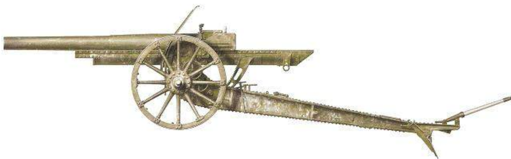
107-мм полевая пушка образца 1910 года. Разрабатывалась и изготавливалась для России французской фирмой «Шнейдер». Артсистема была оставлена на вооружении Красной Армии. Западный фронт, 50-я армия, декабрь 1941 года. A 107-mm field gun (Model 1910) of Red Army. Western Front, 50th Army, December 1941.
