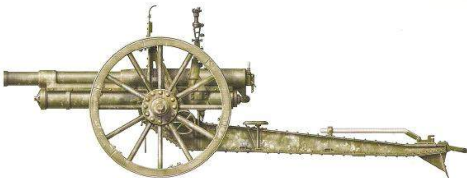
76,2-мм полевая пушка образца 1902 года. Несмотря на то, что представленная конструкция была разработана в 1906 году (именно тогда появилось щитовое прикрытие и панорамный оптический прицел), «трехдюймовки» состояли на вооружении Красной Армии. Западный фронт, 413-я стрелковая дивизия, ноябрь 1941 года. A 76,2-mm field gun (Model 1902) of Red Army. Western Front, 413th Rifle Division, November 1941.
