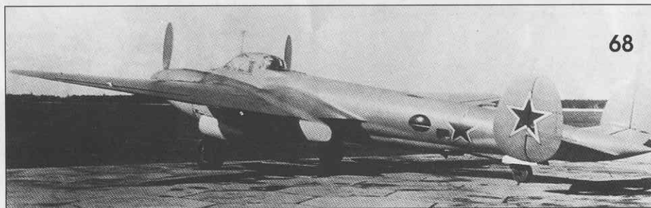
67, 68. Самолет Пе-2М. Хорошо видны верхняя и нижняя установки пушек УБ-20. The Pe-2M. These photos give a good view of the upper and lower UB-20 cannon installations.
