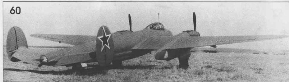
60, 61. Пе-2И мог служить эталоном красоты и чистоты аэродинамических форм. Перед бомбоотсеком видна головка оптического прицела-перископа ОПСК. The Pe-2I showed the evolving beauty and clean form of the design. Just in front of the bomb racks is the sight head for the OPSK periscopic optical bombsight.
