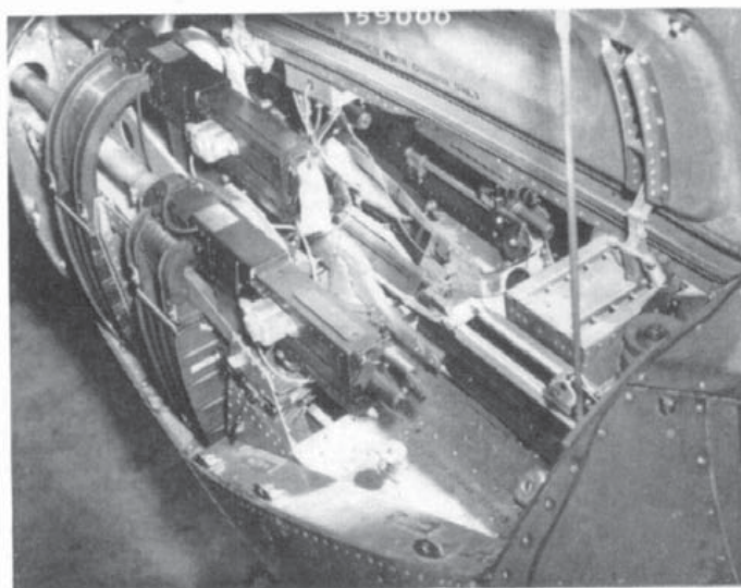
Armament bay of P-38L-5-LO.
