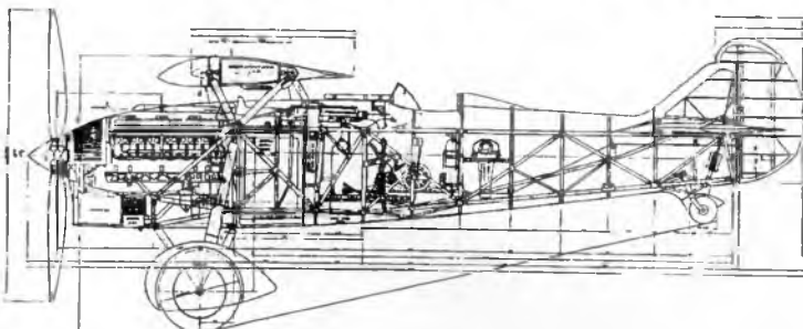
Компановочная схема истребителя Fiat CR.32
