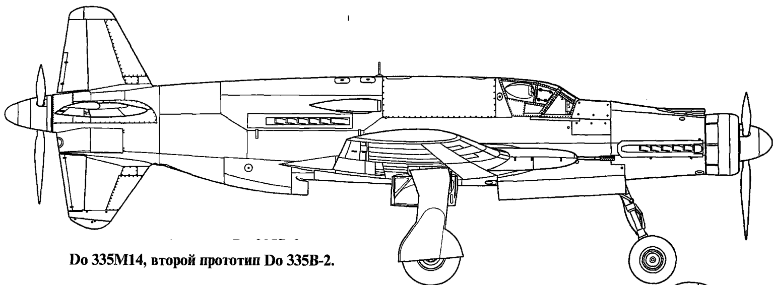
Учебный Do 335B-5 с двигателями Jumo 213. Проект, реконструкция.
