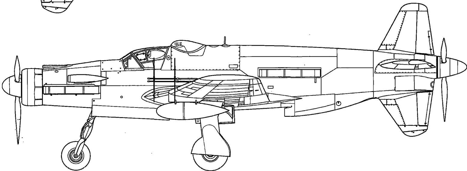
Do 335B-7, вид сбоку, фрагмент крыла. Проект, реконструкция.
