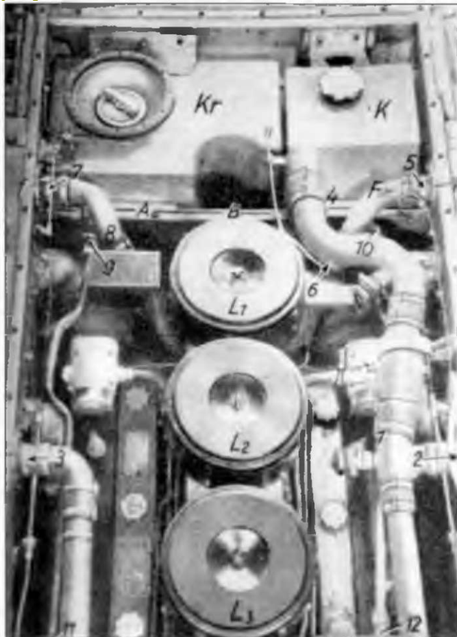
На первых 250 построенных танках «Пантера» Ausf. D были установлены двигатели Майбах HL-210 P30. Небольшой топливный бак (Kr) снабжен полукруглым вырезом под телескопическую трубу воздухозаборника, бак радиатора – К.
