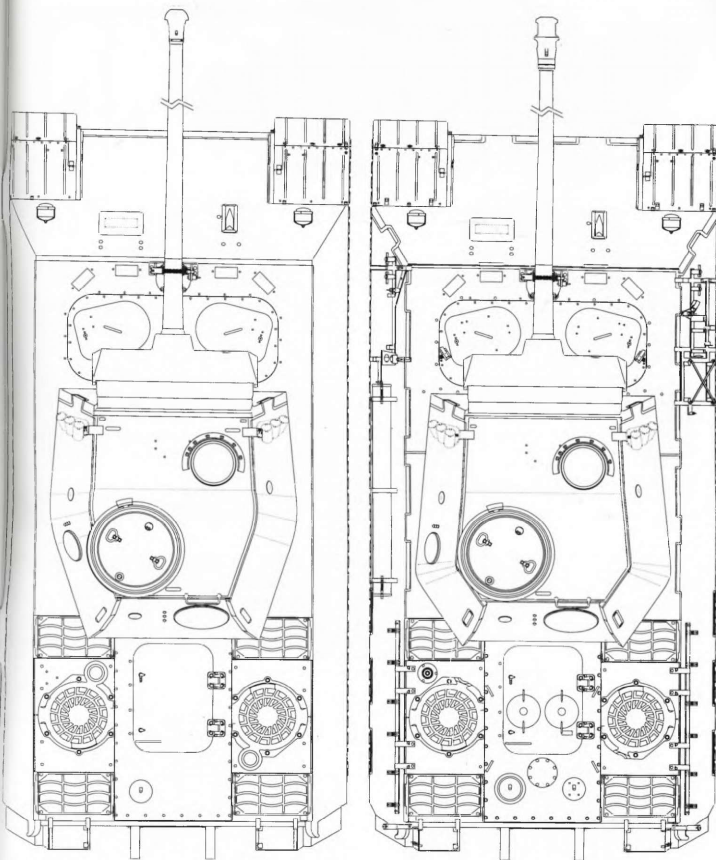
Сравнение опытной машины Fgst.Nr.V2 (слева) и первого серийного танка «Патера» Ausf. D (справа)
