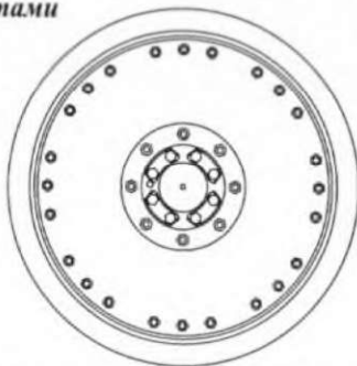
Экспериментальный опорный каток с восьмью группами по три болта в каждой
