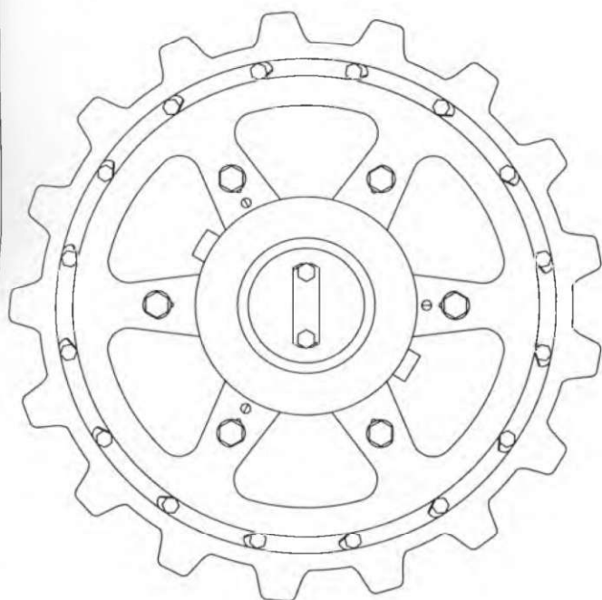
Ведущее колесо с 16 болтами и 16 шплинтами
