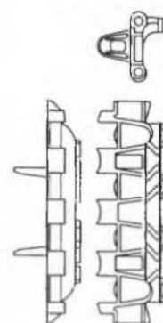
Шесть шевронов (Gleitschutzpickeln) высотой 15 мм на траке Kgs-64/660/150
