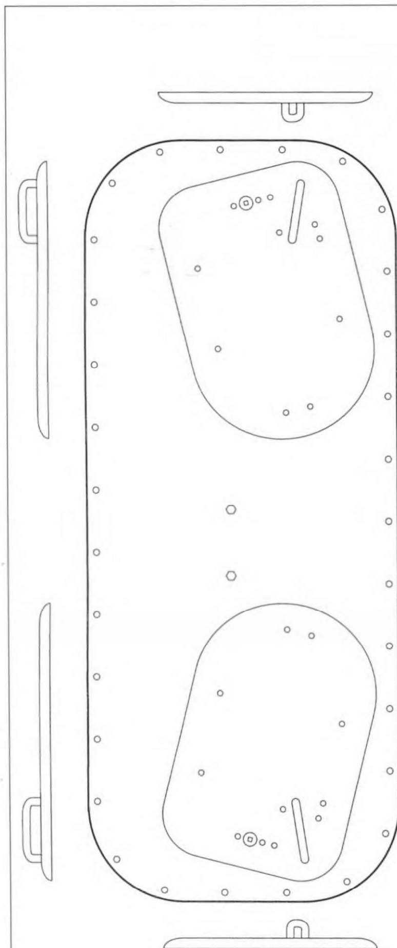
Ручки на люках стрелка-радиста и механика-водителя
