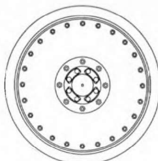
Опорный каток с 24 болтами
