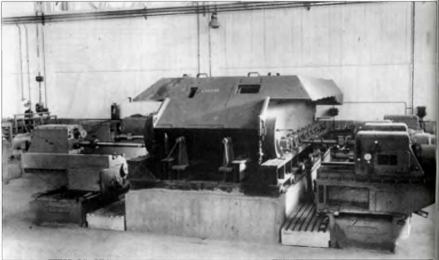
В противовес слухам о толщине лобового листа корпуса «Пантеры» Ausf. D в 60 мм, снимки Wanne Nr 210006 и 210010 показывают, что толщина брони составляла 80 мм. В сравнении с шасси Fgst.Nr. V2 передний перископ механика-водителя смещен примерно на 490 мм от продольной оси.
