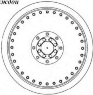
Экспериментальный опорный каток с 32 крепежными болтами
