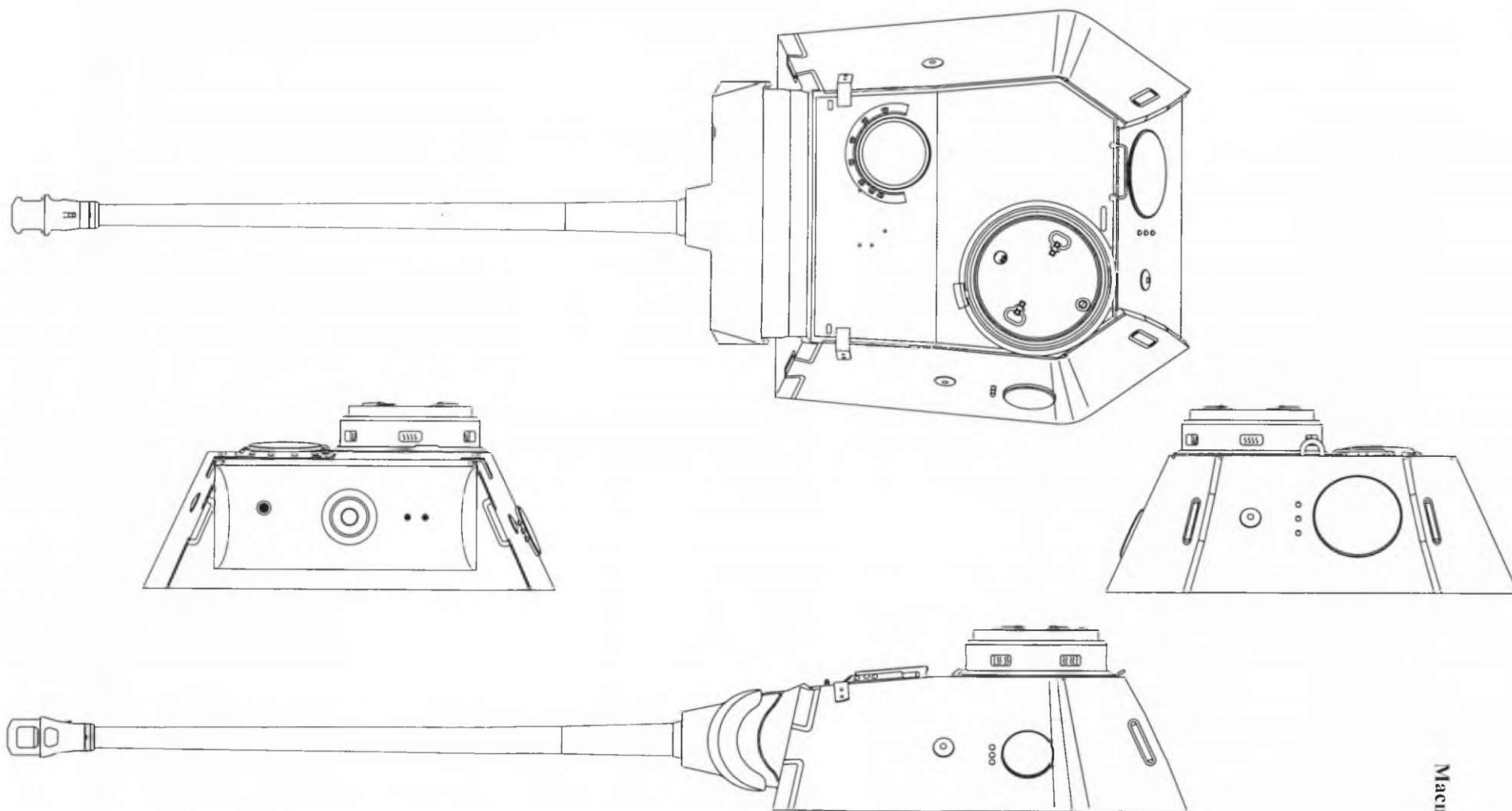
Башня в сборе перед монтажом на шасси танка Pz.Kpfw. Panther Ausf. D. Все отличия первых серийных башен сборки января 1943 г. со сдвижным командирским люком на штыре, расположенном сзади слева
