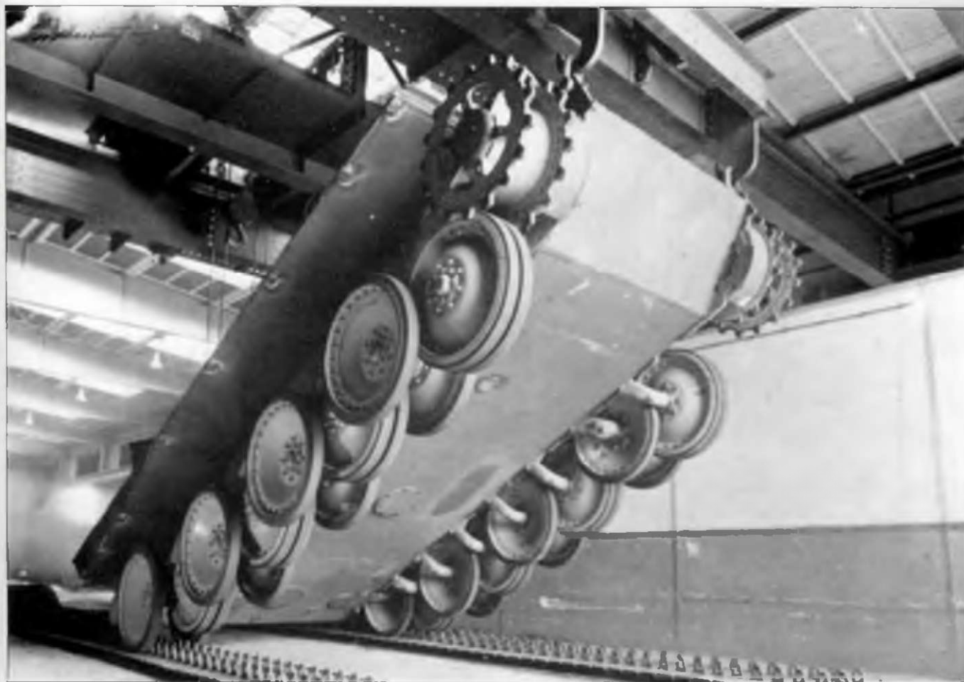
«Пантера» Ausf. D постройки августа 1943 г. все еще имеет цельное днище толщиной 16 мм! Опорные катки – усиленные, с 24 болтами каждый. На нижней поверхности надгусеничной полки приварен только один кронштейн крепления бортового экрана. На лицевой поверхности траков Kgs. 64/660/150 отлиты шевроны.
