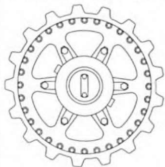
Усиленное ведущее колесо с 32 контрольными болтами и гайками с проволоочными шплинтами
