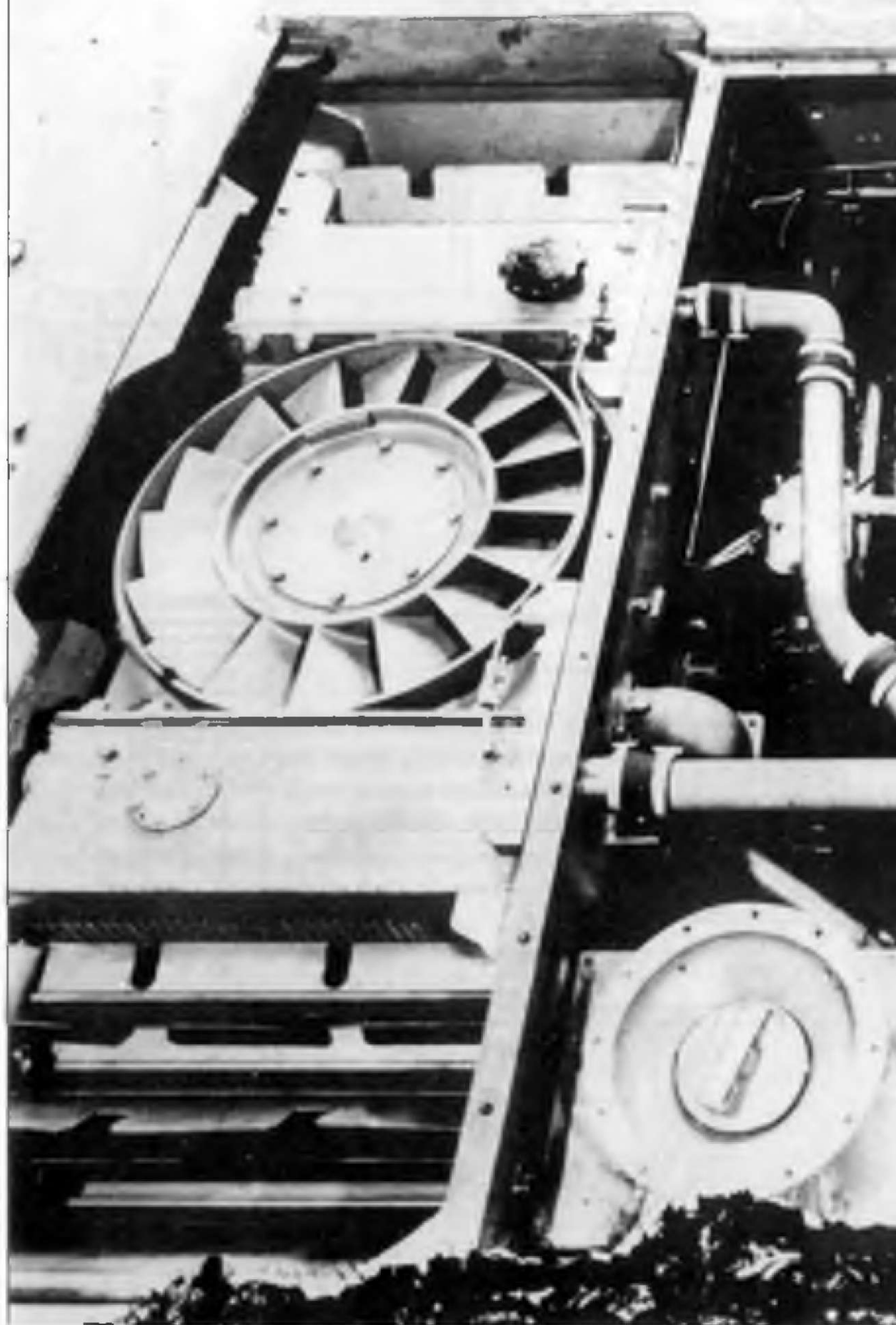
Моторное отделение шасси Fgst.Nr. V2 (не серийной «Пантеры») с большим топливным баком в кормовой части и заливочными горловинами радиаторов.
