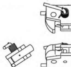
Замок, предотвращающие сдвиг люка механика-водителя
