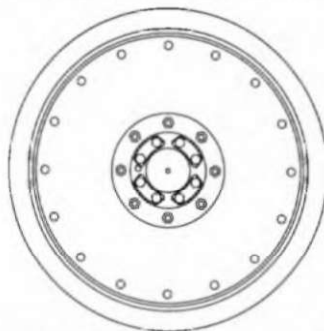
Экспериментальный опорный каток с 16 заклепками или 16 болтами
