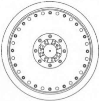
Модернизированный усиленный опорный каток с 16 заклепками
