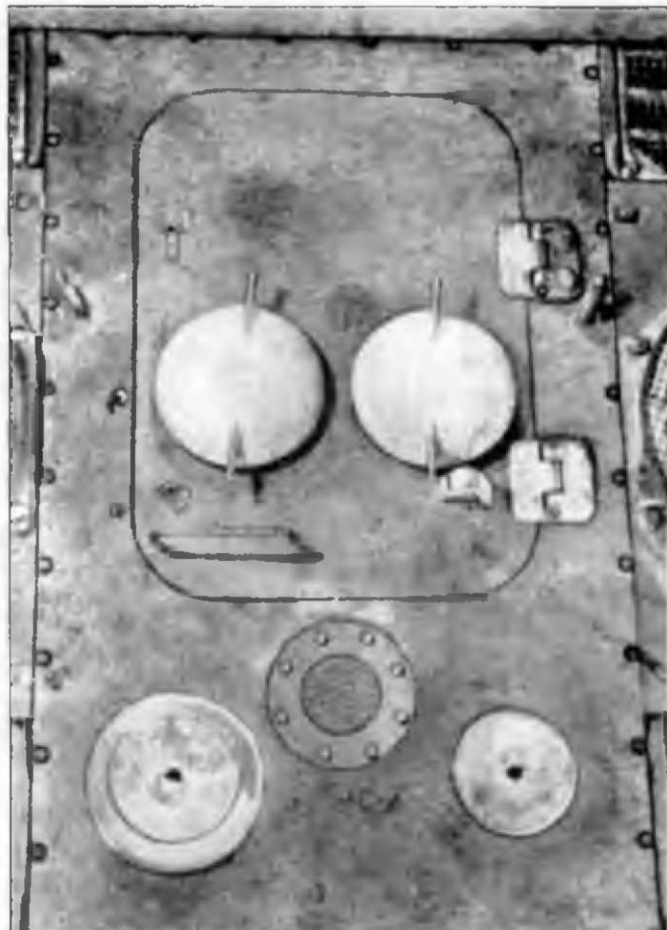
Крышка моторного отделения «Пантеры» Ausf. D с «вилками», приваренными в бронекорпусам воздухозаборника, крышки топливного бака и бака радиатора и заглушки воздухозаборника-иниорхеля раннего типа.
