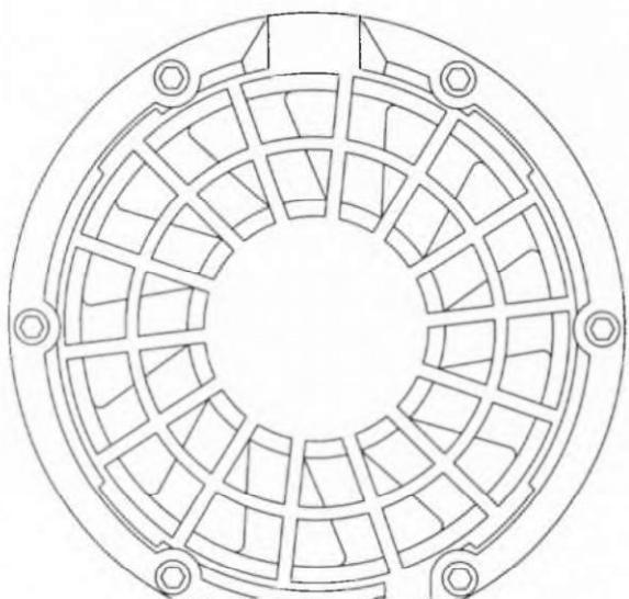
Доработанная литая бронедеталь с круглым основанием
