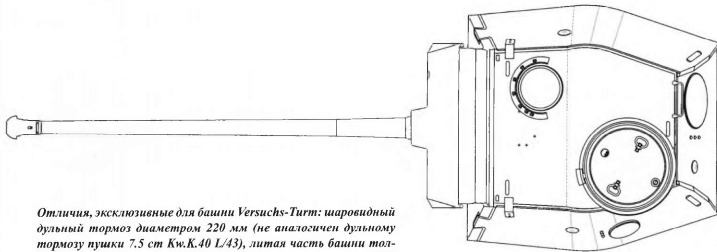
Panzerkampfwagen "Panther", башня Versuchs-Turm, установленная на шасси Fgst.Nr.V2
