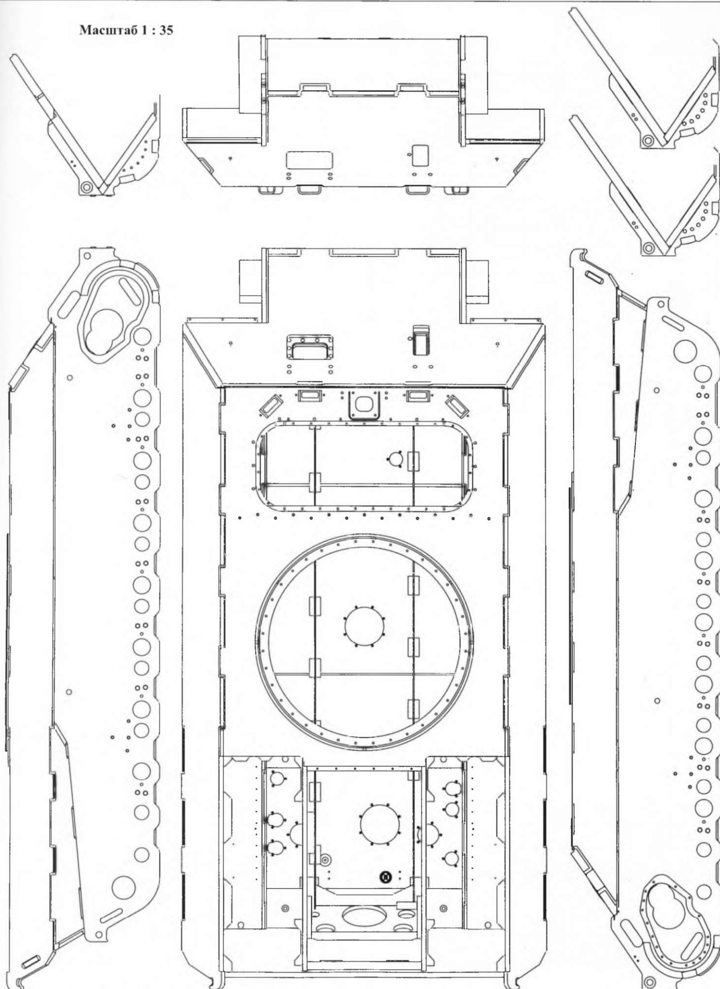
Корпус танка Panzerkampfwagen "Panther" Ausf. D в том виде, в каком он поставлялся на завод окончательной сборки от производителя
