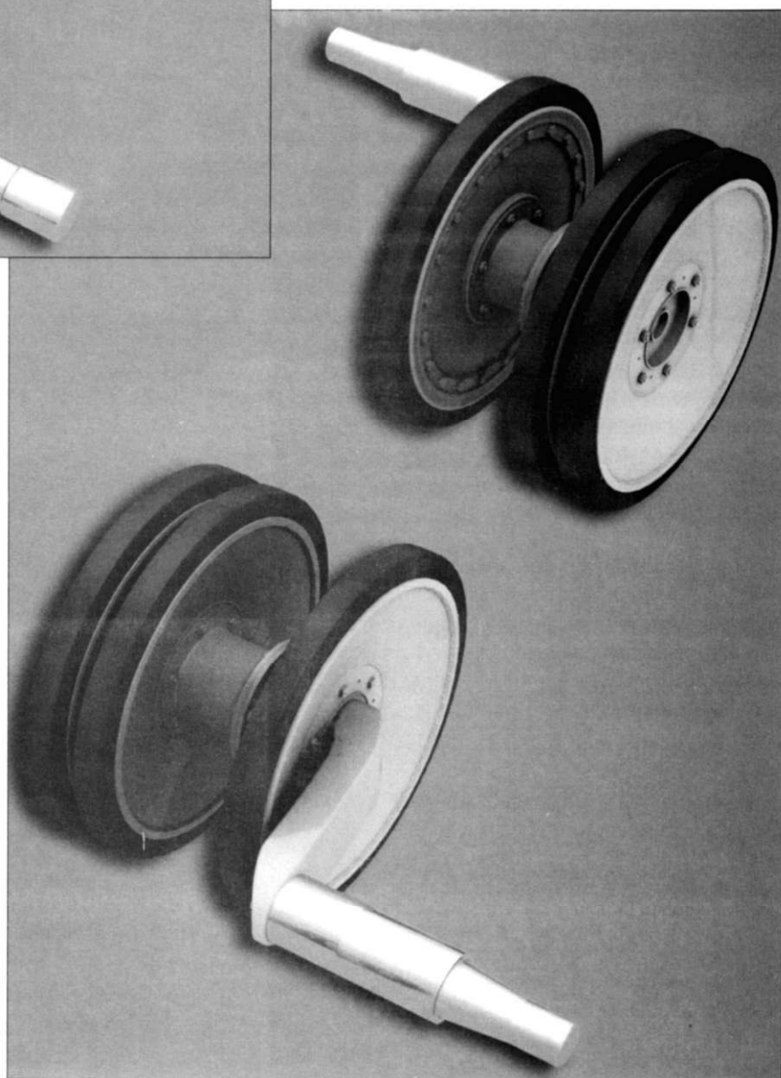
Вид снаружи и изнутри на первый опорный каток с подвеской и торсионам. Торсионы первого и последнего опорных катков имели больший диаметр, чем стальных.
