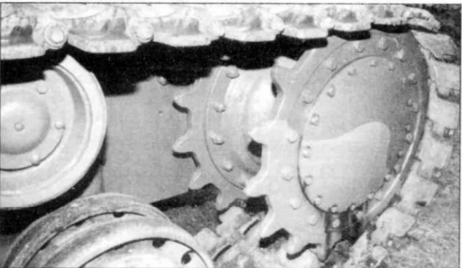
Ведущее колесо, опорный каток и поддерживающий ролик образца 1940 г.
