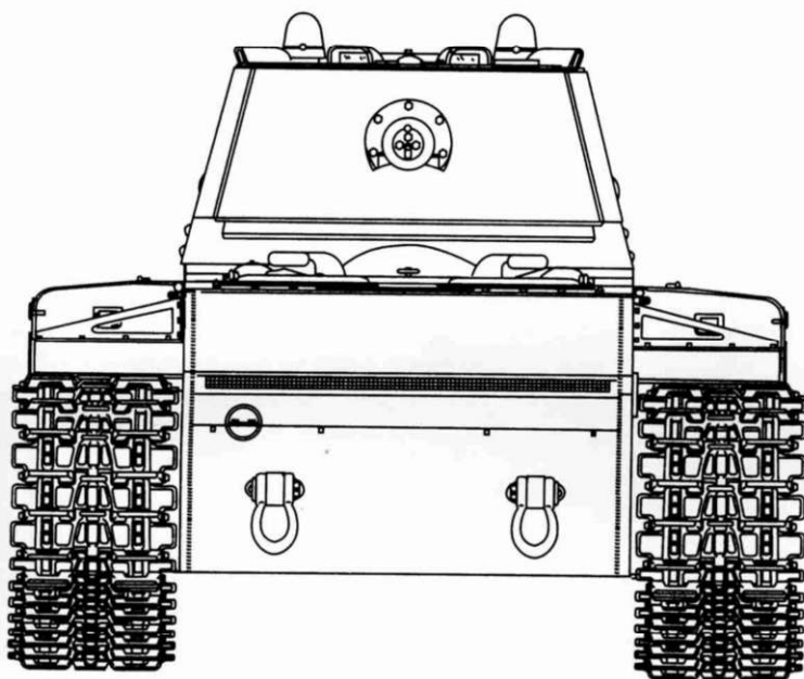
КВ-1 проекта 1940 г. ЛКЗ ранних производственных серий. Вид сзади.
