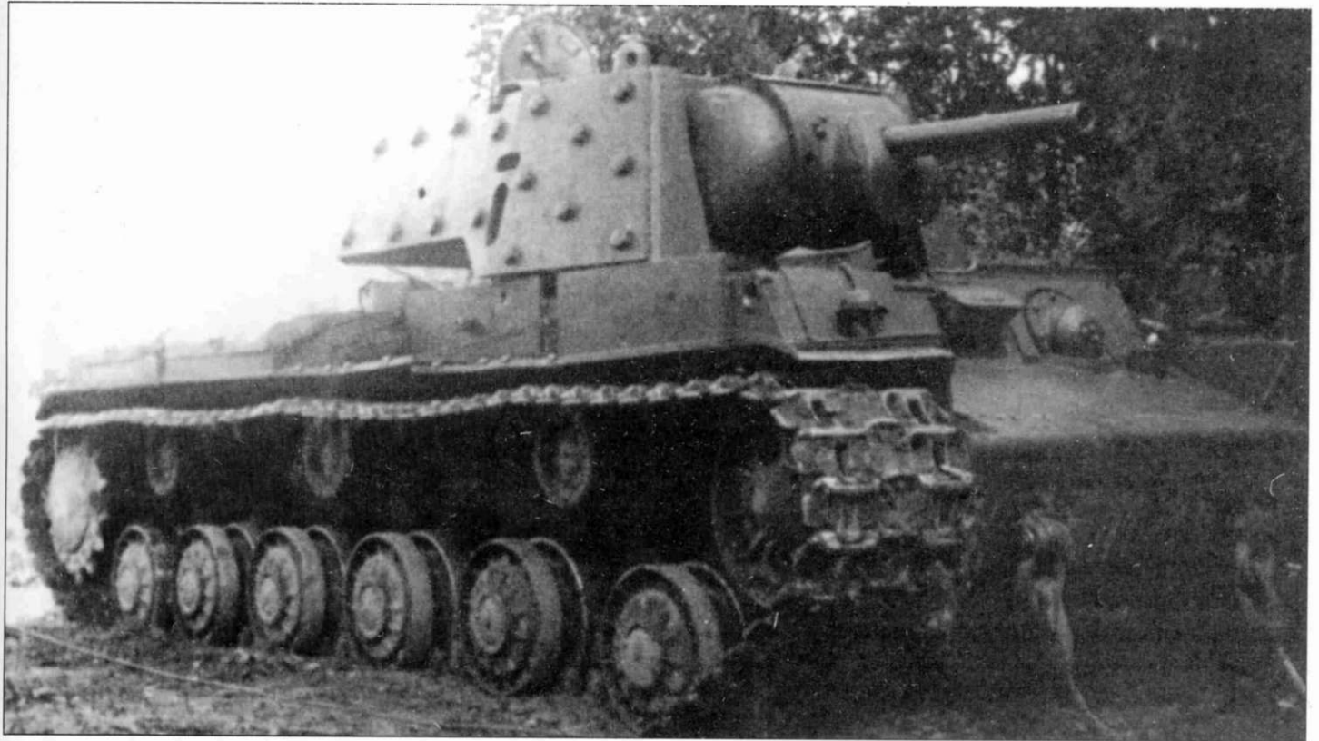
Редкий фотоснимок, на котором запечатлен танк КВ-1 проекта 1940 г. поздних производственных серий (с дополнительными наварными листами брони на корпусе) с экранами. Различие между ранними наварными броневыми листами и более поздними экранами, устанавливаемыми на корпусе в районе башенного погона становится ясным при сравнении этой фотографии с фотографией ниже.
