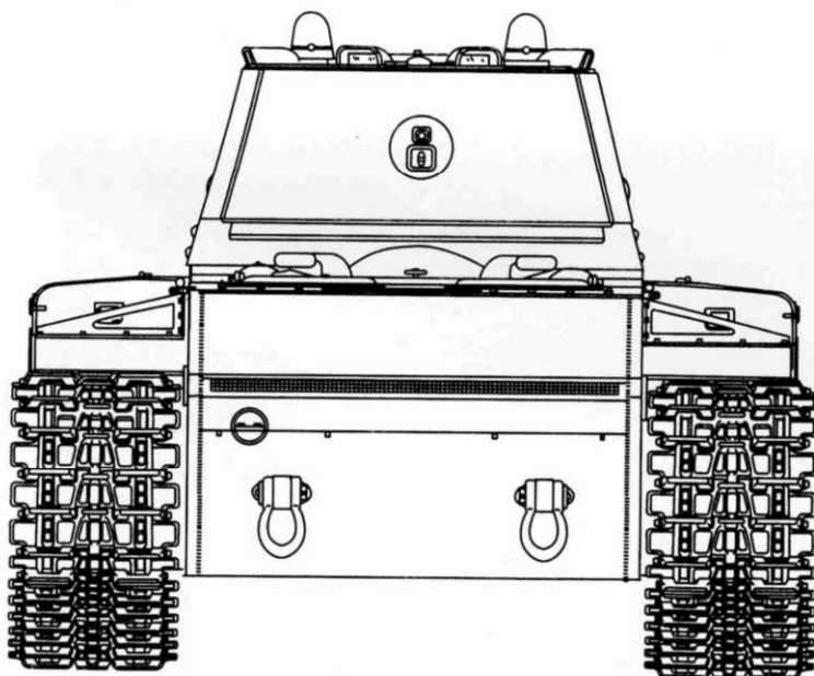
КВ-1 проекта 1939 г. ЛКЗ, ранних производственных серий. Вид сзади.
