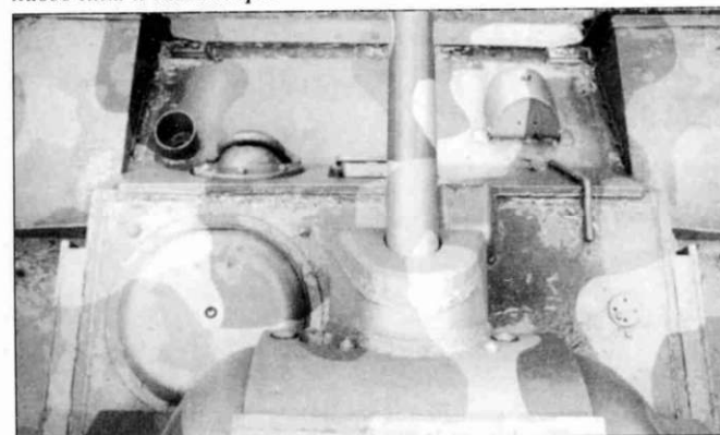
Передняя часть башни с бронированной крышкой вентилятора, перископическим прицелом наводчика (ПТ-4-7) впереди слева и перископом командира танка (ПТК) впереди справа. Позади них бронированные крышки неподвижных приборов наблюдения наводчика и командира.
