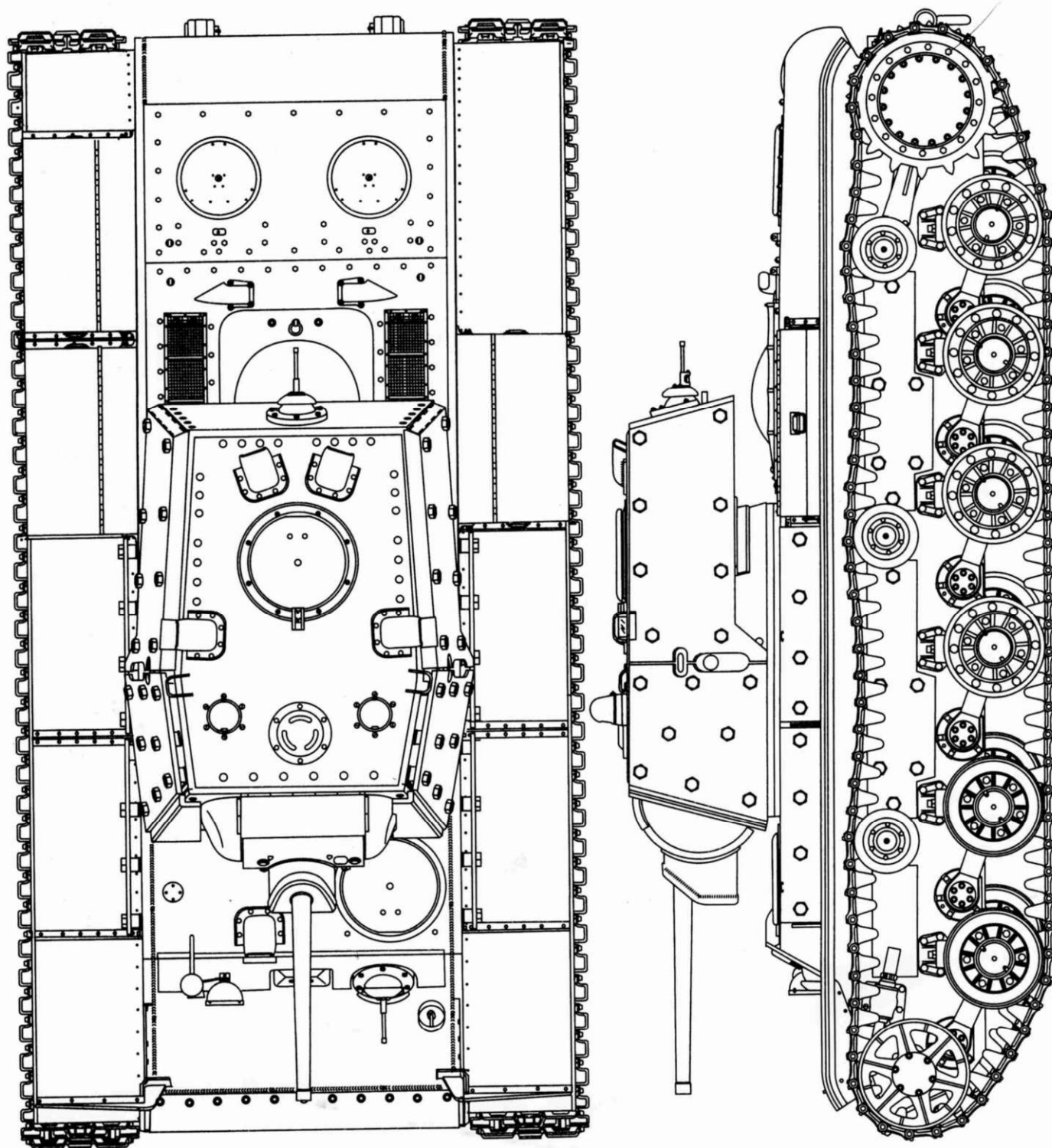
КВ-1 проекта 1940 г. поздних производственных серий с экранами (на корпусе и башне). Вид сверху и сбоку.
