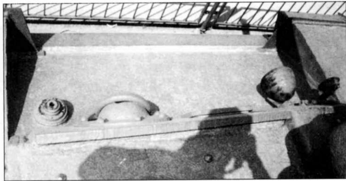
Вид сверху на передний лист корпуса с креплением шаровой установки пулемета. Видна дополнительная броневая плита установленная на корпусе. В правой части фотографии видна фара, а в левой - антенный ввод.
