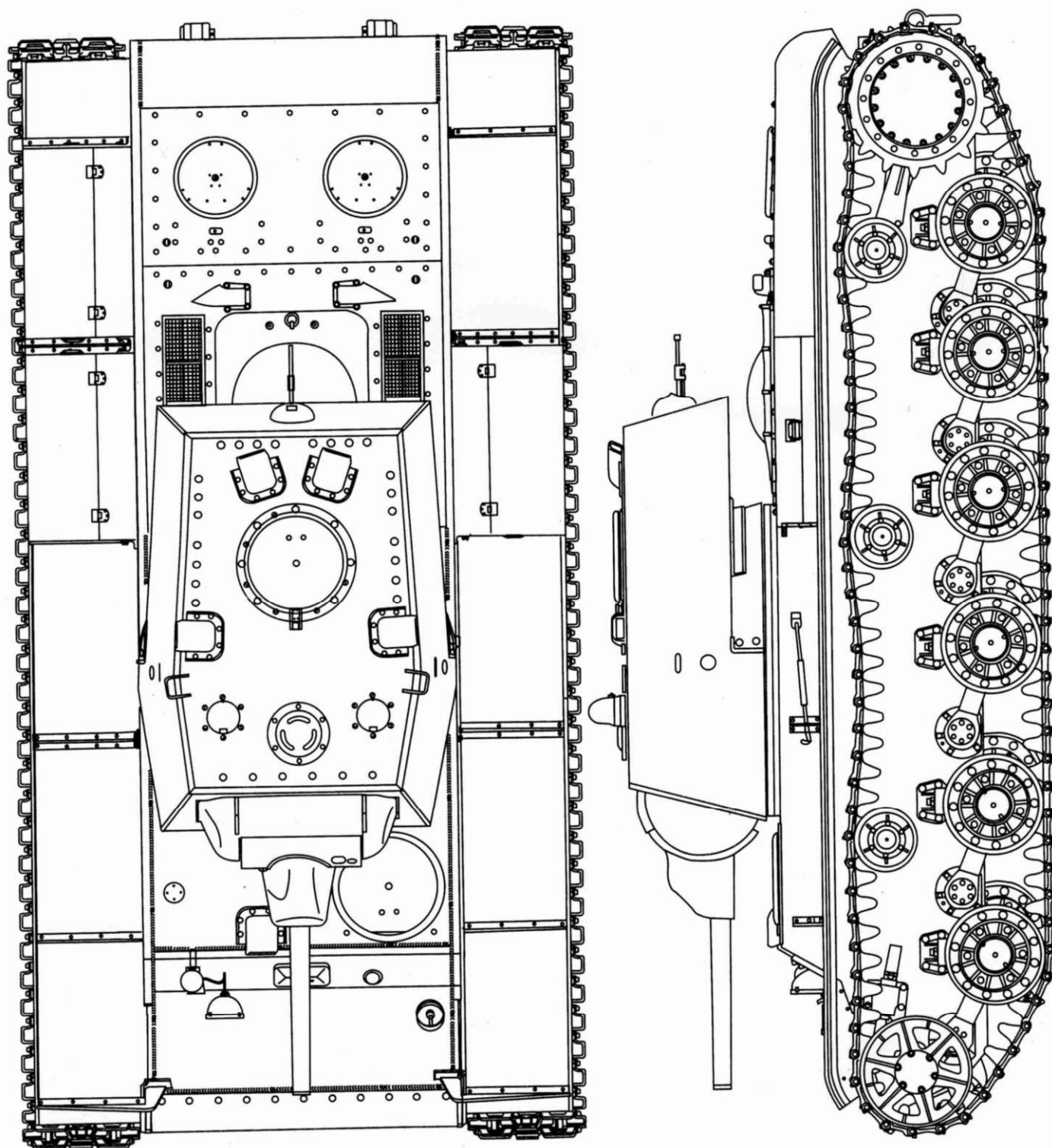
КВ-1 проекта 1939 г. ЛКЗ, ранних производственных серий. Вид сверху и сбоку.
