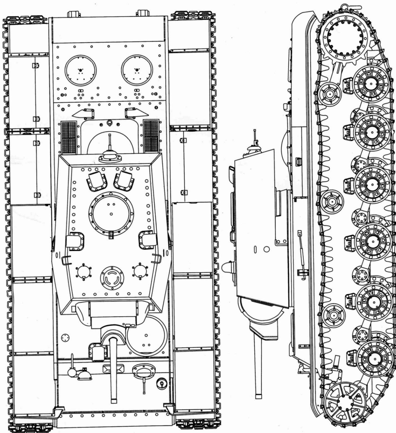
КВ-1 проекта 1940 г. ЛКЗ, ранних производственных серий. Вид сверху и сбоку.
