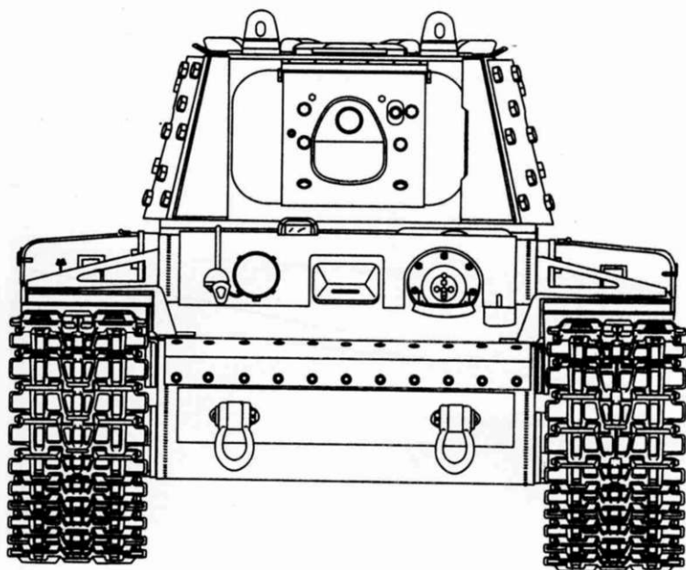
КВ-1 проекта 1940 г., поздних производственных серий с экранами (на корпусе и башне). Вид спереди и сзади.
