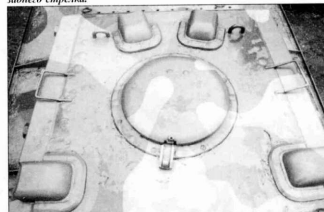
Задняя часть крыши башни с башенным люком и креплением для зенитного пулемета. На переднем плане снова неподвижные приборы наблюдения командира и наводчика, а на заднем плане видны два прибора наблюдения заднего стрелка. Толщина деталей экранов производит впечатление.
