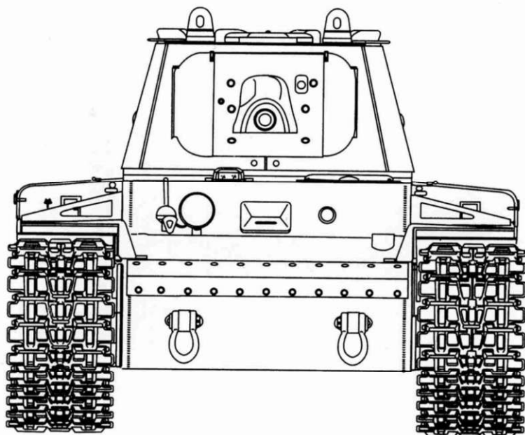
КВ-1 проекта 1939 г. ЛКЗ, ранних производственных серий. Вид спереди.
