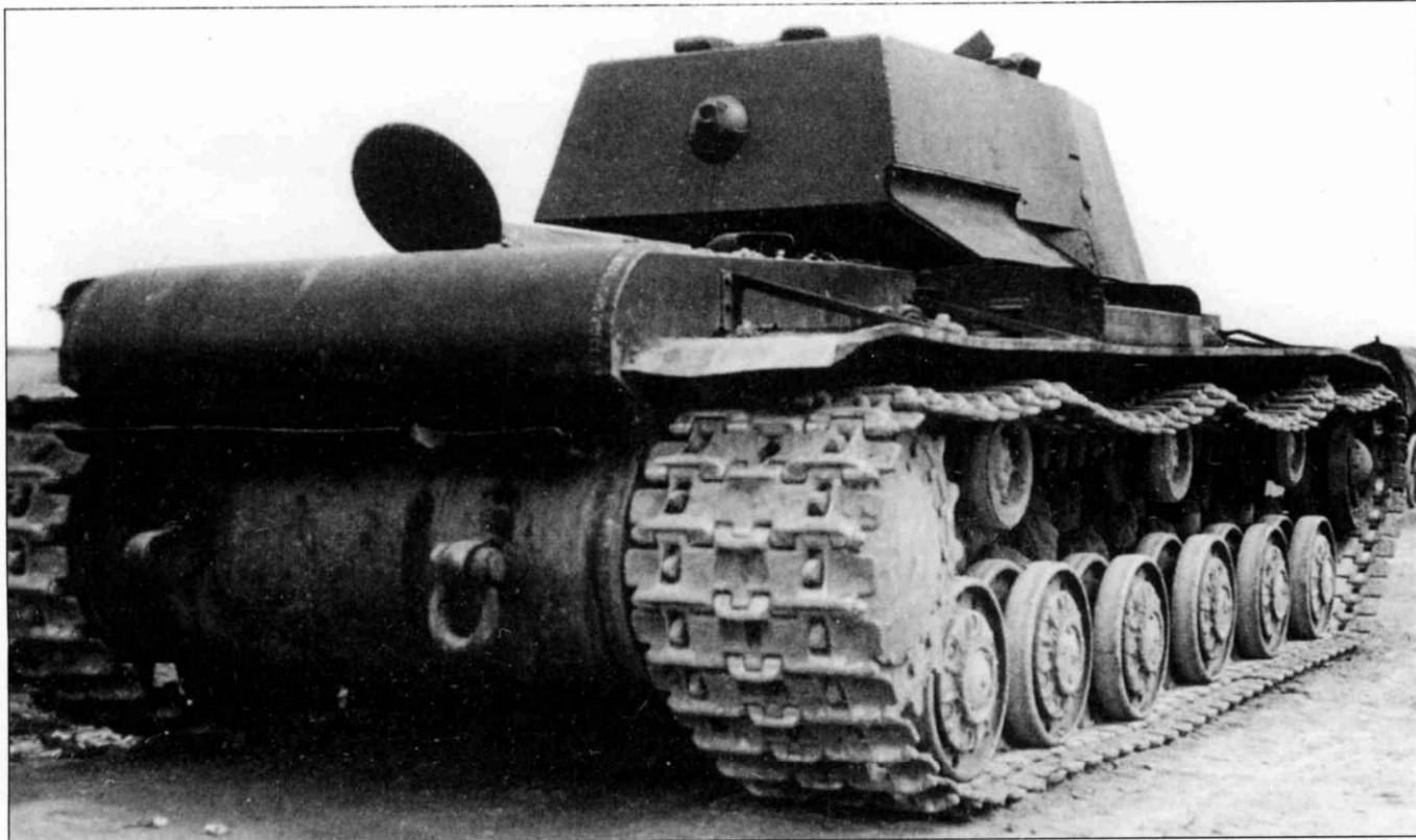
КВ-1 проекта 1939 г., вид сзади. Обратите внимание на конструкцию крепления шаровой установки кормового башенного пулемета раннего типа без бронированного фланца.
