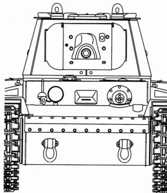
КВ-1 проекта 1939 г. ЛКЗ, поздних производственных серий. Вид спереди.
