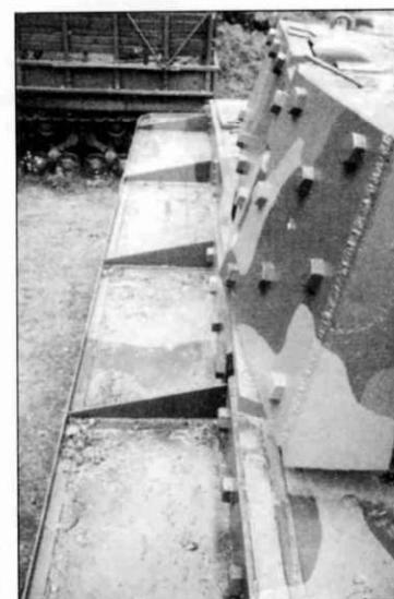
Передняя часть боевого отделения, в которой располагались механик-водитель (справа) и стрелок-радист (слева). Обратите внимание на ограждение фары - это финская модификация.
