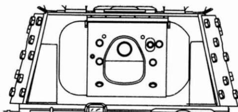
Один из вариантов переднего дополнительного бронирования башни.
