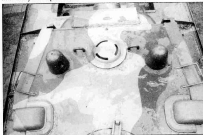
Передняя часть башни с бронированной крышкой вентилятора, перископическим прицелом наводчика (ПТ-4-7) впереди слева и перископом командира танка (ПТК) впереди справа. Позади них бронированные крышки неподвижных приборов наблюдения наводчика и командира.
