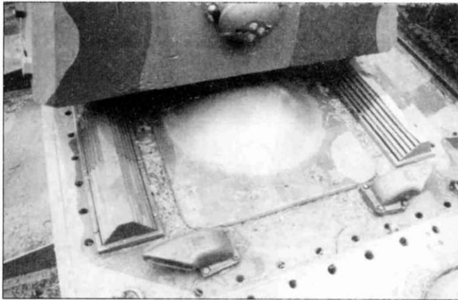
Большой люк для доступа к двигателю, частично прикрытый кормой башни, и выхлопные патрубки. На экспонируемом танке в этом месте отсутствует значительное количество болтов.
