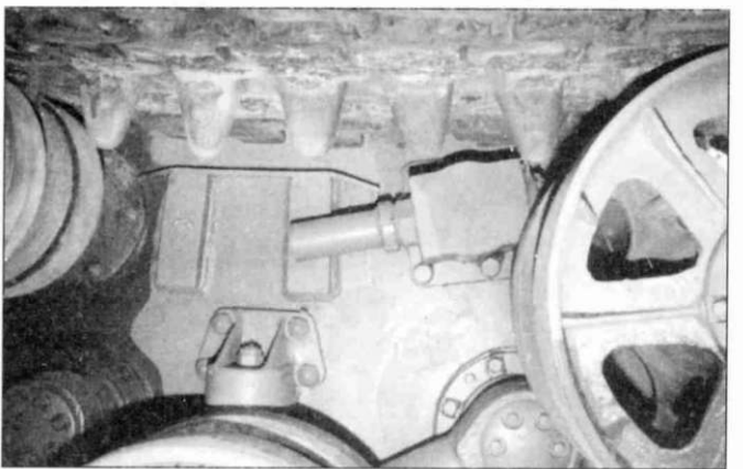
Упор балансиров и механизм натяжения гусеницы за ленивцев.
