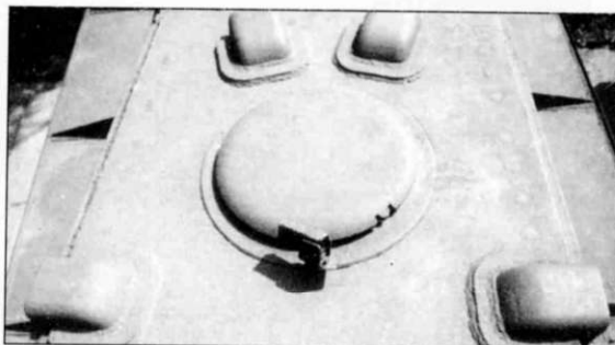
Задняя часть крыши башни с посадочным люком и креплением для установки зенитного пулемета. Впереди видны неподвижные перископы командира и наводчика, а сзади - два неподвижных перископа стрелка кормового пулемета.
