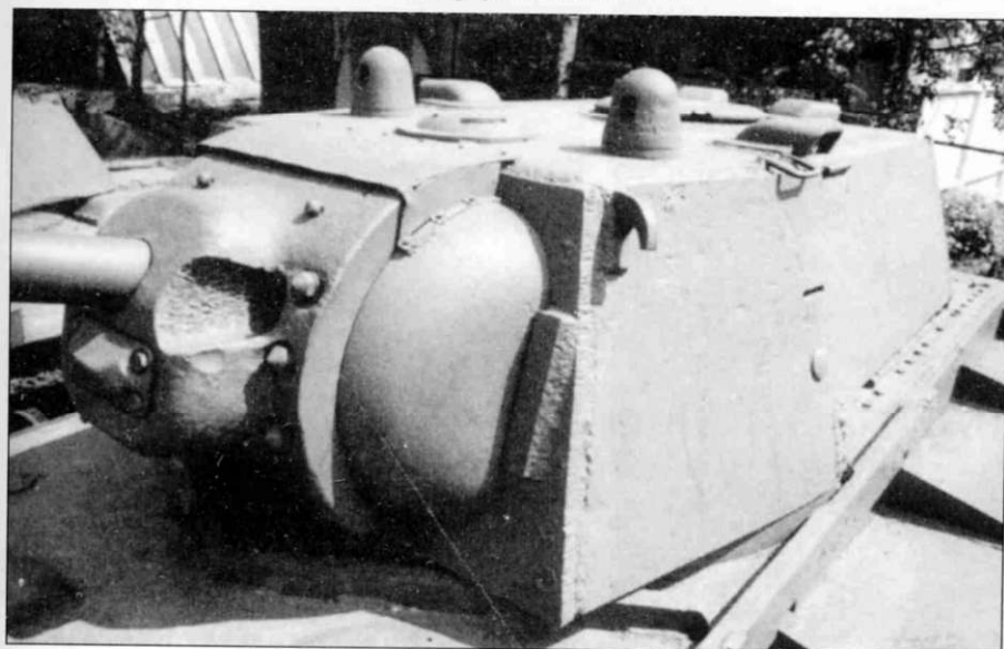
Вид башни спереди. Виден небольшой лючок для обслуживания 76,2 мм пушки ЗиС-5 и типичный вырез в маске пушки. Крюков для подъема башни на серийных машинах не было, они приварены позже во время испытаний.
