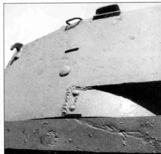
Левая сторона башни с амбразурой для стрельбы из личного оружия и смотровой щелью наводчика со стеклоблоком. Такая же щель имеется и на правой стороне башни для командира танка.
