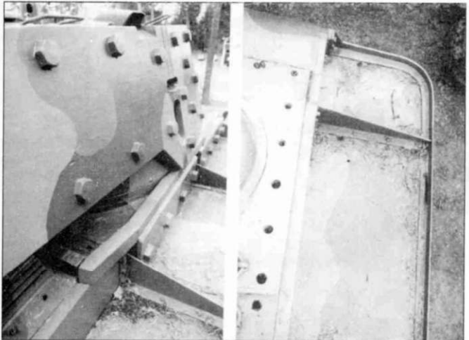
Три снимка надгусеничных полок в районе башни и моторно-трансмиссионного отделения. Еще раз обратите внимание на толщину броневых листов.
