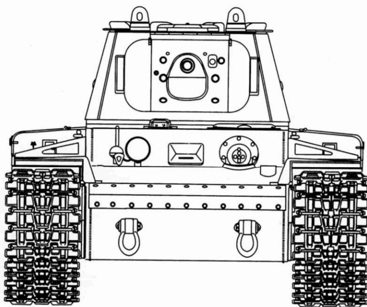
КВ-1 проекта 1940 г. ЛКЗ ранних производственных серий. Вид спереди
