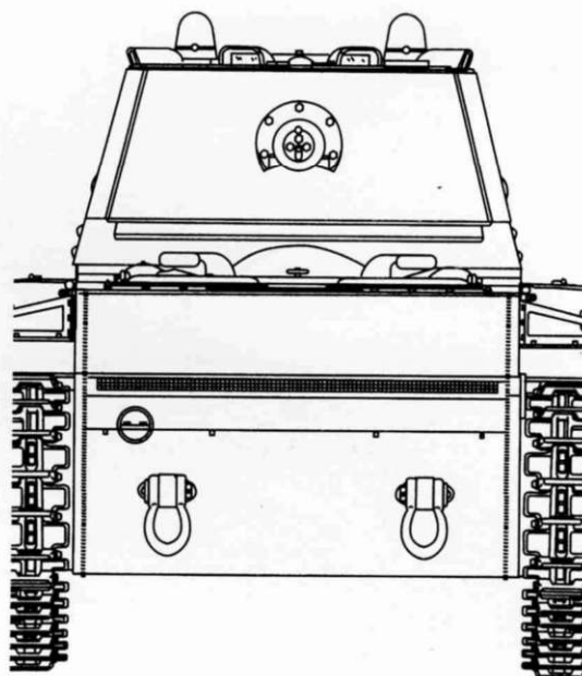
КВ-1 проекта 1939 г. ЛКЗ, поздних производственных серий. Вид сзади.
