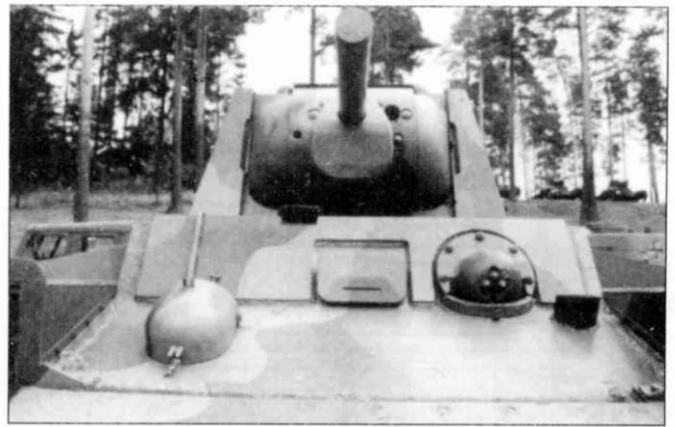
Вид спереди демонстрирует детали передних листов корпуса, здесь виден дополнительный приваренный броневой лист перед местом механика-водителя и финское ограждение фары. Обратите внимание также на бронировку орудийной маски.
