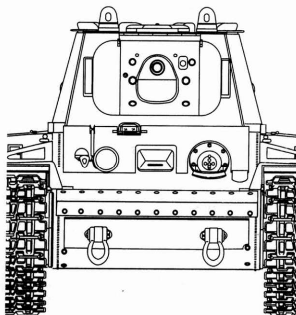
КВ-1 проекта 1940 г. ЛКЗ поздних производственных серий. Вид спереди и сбоку.
