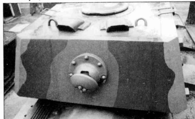
Корма башни, хорошо видно крепление шаровой установки пулемета ДТ, калибра 7,62 мм. На крыше башни два прибора наблюдения заднего стрелка.
