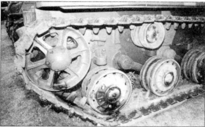
Детали ленивца, передняя часть корпуса.
