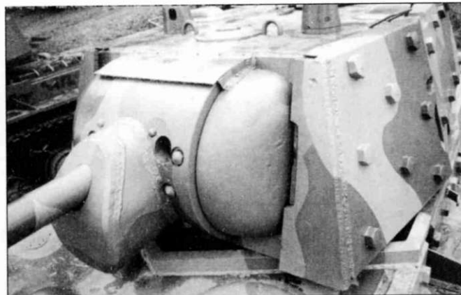
Левая сторона маски пушки Ф-32 с отверстием под телескопический прицел наводчика ТМФД.
