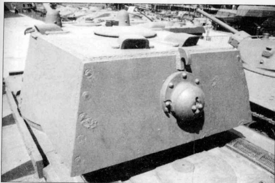
Тыльная часть башни с креплением шаровой установки для 7,62 мм пулемета. Обратите внимание на крепление кормового листа башни. Соединение было или болтовым, или сварным или комбинированным, в зависимости от завода изготовителя. Здесь хорошо видна толщина дополнительных листов бронирования по бортам корпуса.
