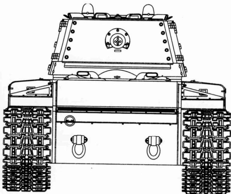
КВ-1 проекта 1940 г., поздних производственных серий с экранами (на корпусе и башне). Вид спереди и сзади.
