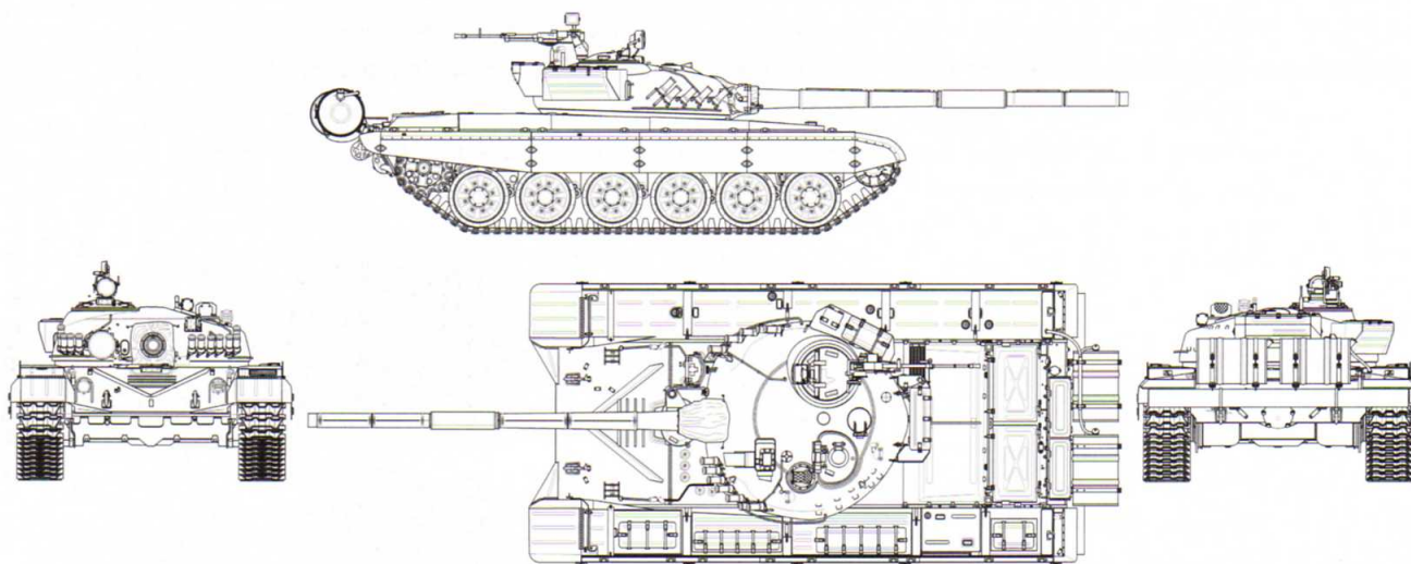
Т-72А. Вид справа, спереди, сверху, с кормы.
