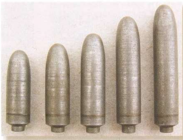
■ Обнаруженные в 1970-е годы 9-мм реактивные пули с ведущим медным пояском разработки Шурка, D.W.M.
