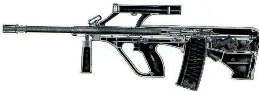
■ Схема устройства штурмовой винтовки StG-77 (AUG/A1). На пламегаситель надет защитный колпачок
