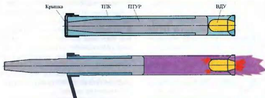
■ Схема запуска ПТУР 9М111 «Фагот»
