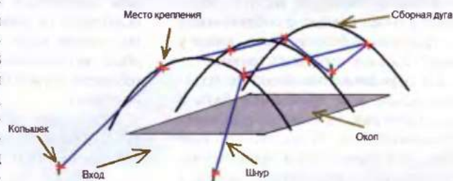
■ Рис. 2. Сборно-разборный «адыгейский домик»
