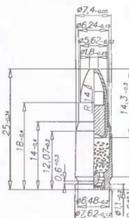
■ Чертеж патрона МПЦ
