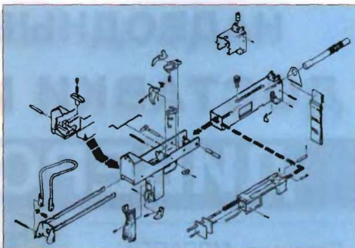
Взрыв-схема M10 «Ингрэм»
