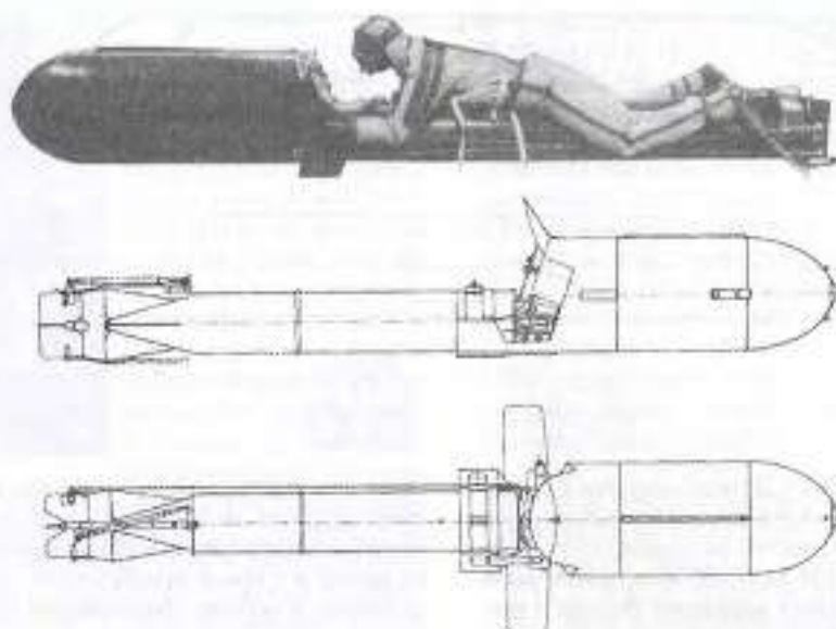
Подводный буксировщик (ПБ) R-1
