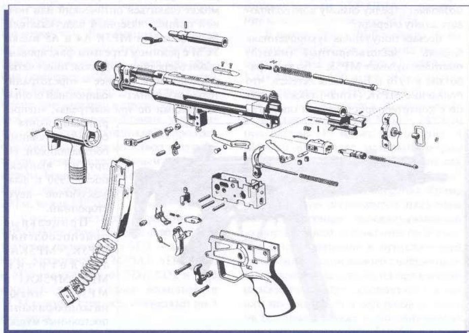
Взрыв-схема пистолета-пулемета MP5K A1
