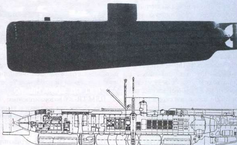
Малая подводная лодка (ПЛМ) MG-110
