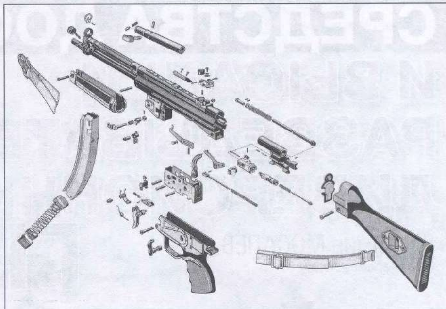
Взрыв-схема пистолета-пулемета MP5A2
