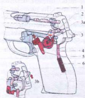
Схема устройства ударно-спускового механизма пистолета P239 «ЗИГ-Зауэр»: 1 — ударник, 2 — шептало, 3 — курок, 3a и 3b — боевой и предохранительный взвод курка, 4 — тяга курка, 5 — рычаг безопасного спуска, 6 — боевая пружина
