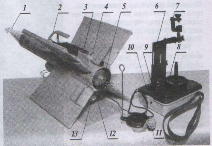
«Кобра» в положении готовности к пуску:
