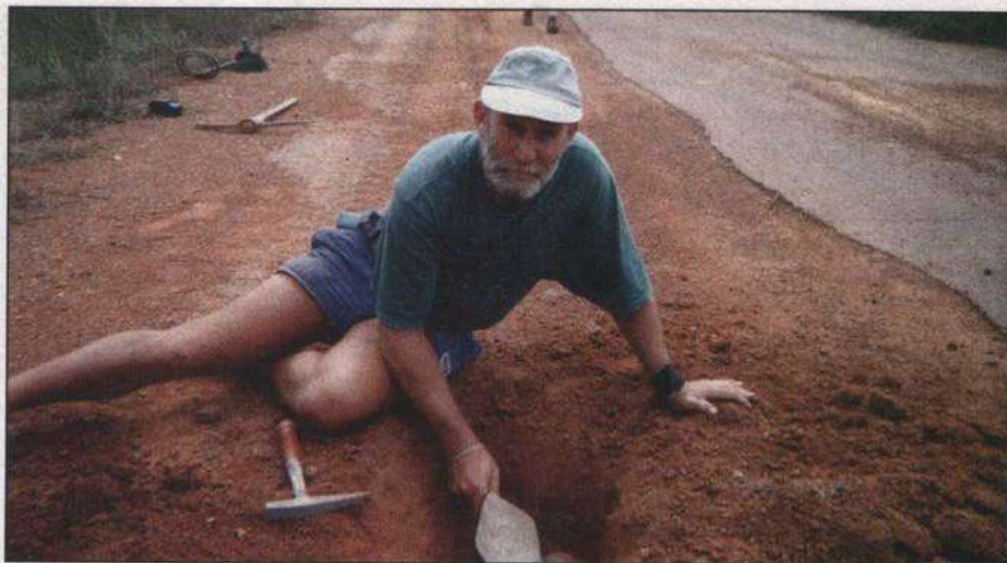
Оператор использует полотенце и геологический молоток для раскапывания китайской противопехотной мины Тип 72, установленной над противотанковой миной
