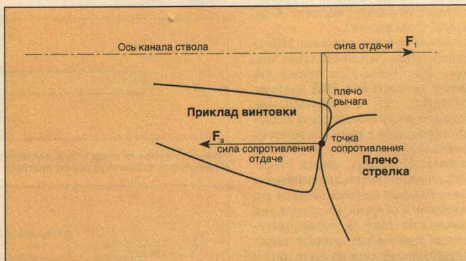
В момент выстрела сила отдачи направлена в плечо. Оно начинает давить на винтовку еще тогда, когда пуля не покинула канал ствола. Сила отдачи направлена выше точки сопротивления. Образуется рычаг сил. Крутящий момент подбрасывает ствол вверх
