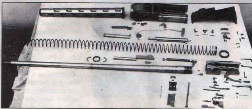
Пулемет Модель 5 калибра 12,7 мм после полной разборки
