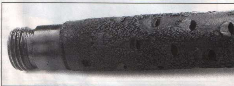
Сильный нагар на наружной поверхности ствола Мк.5 удивительно мало повлиял на эффективность глушителя
