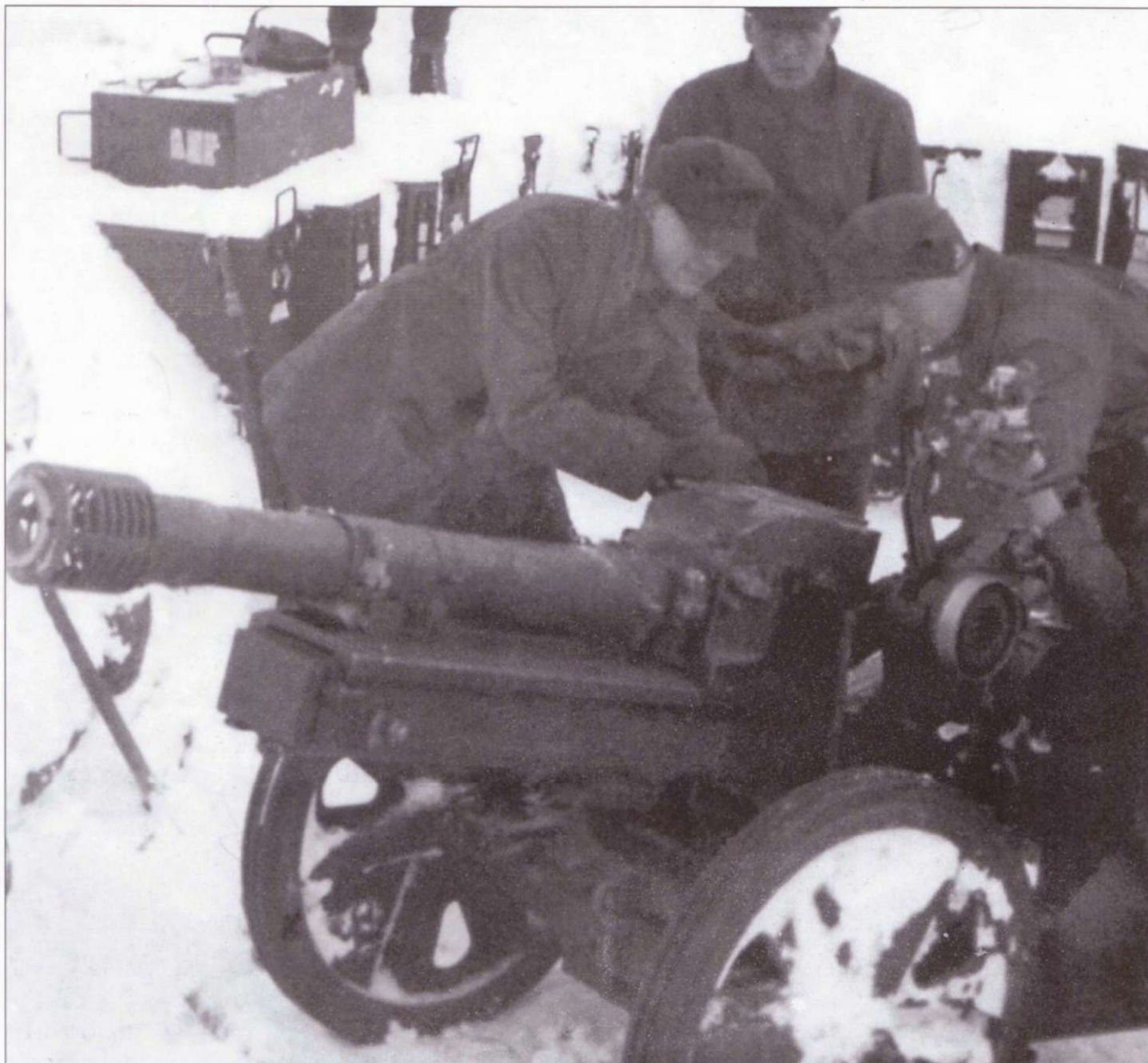
75-мм горная пушка на огневой позиции в горах. Рядом уложены ящики с боеприпасами, которые образуют своего рода стенку, защищающую пушку от осыпающегося снега - позиция отрыта в сугробе. При стрельбе в горах не всегда удавалось точно определить требуемый угол возвышения орудия по причине резкого перепада высот между огневой позицией и целью. Точность стрельбы падала.
