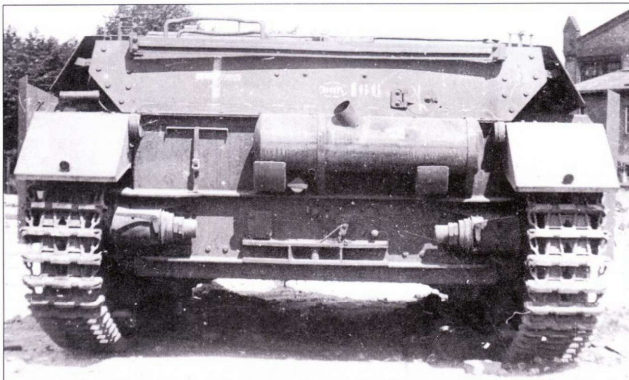
Кормовая часть ранних Jagdpanzer IV/70(V).
