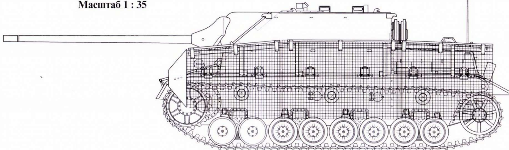
Jagdpanzer IV/70(A) с двумя катками с внутренней амортизацией и сетчатыми экранами
