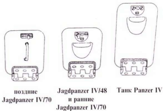
Люки доступа к тормозам
