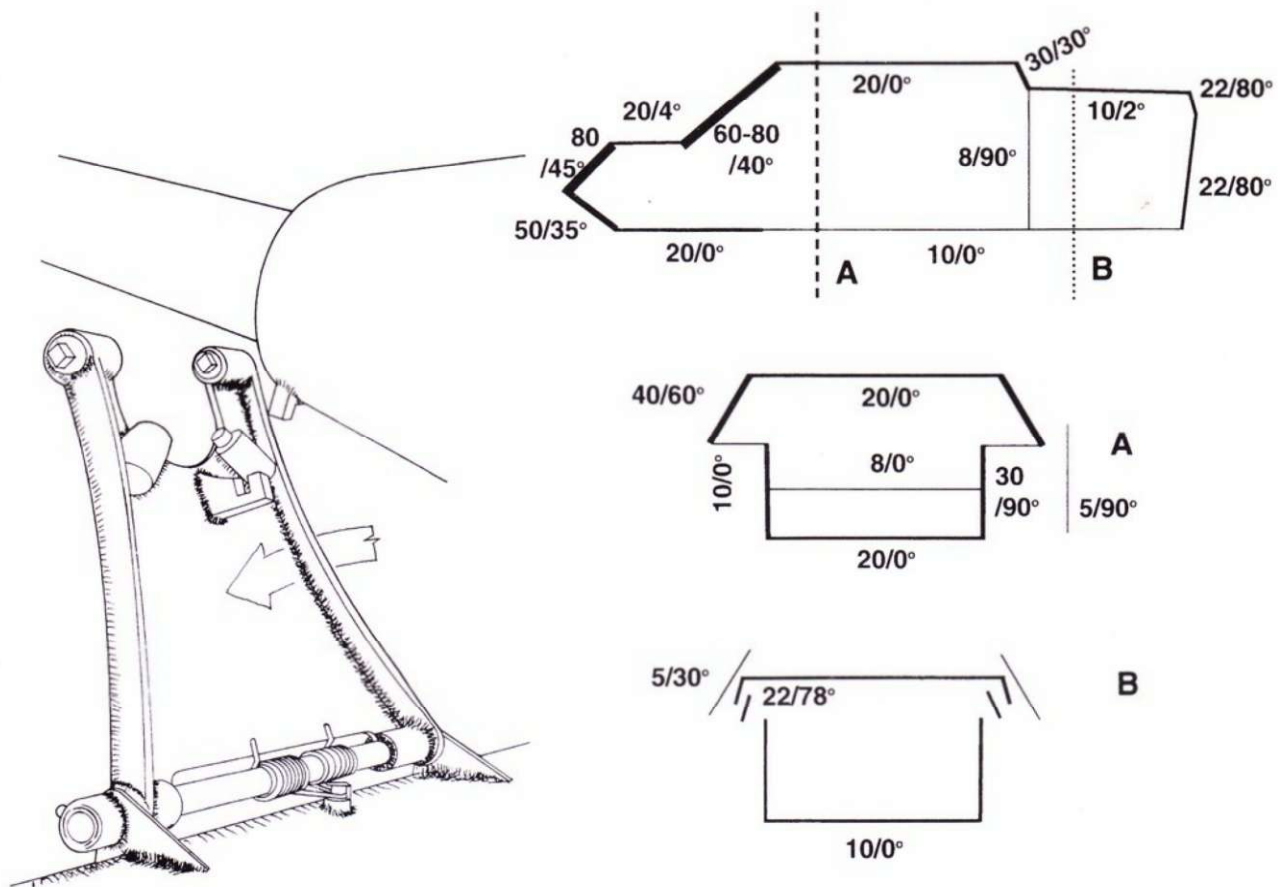
Схема бронирования Jagdpanzer IV/70
