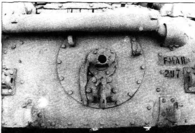
Отверстие под ручной стартер. Место выхода выхлопного патрубка из корпуса закрыто бронеклаком. Абердин.
