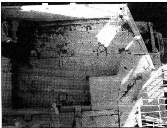
Люк доступа к двигателю одновременно является полом боевого отделения, Абердин.
