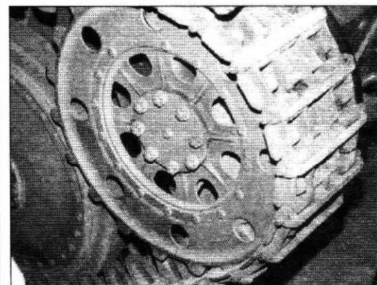
Детализовка правого ведущего колеса. Истребитель танков Sd.Kfz. 139 из музея в Самюре, Франция.
