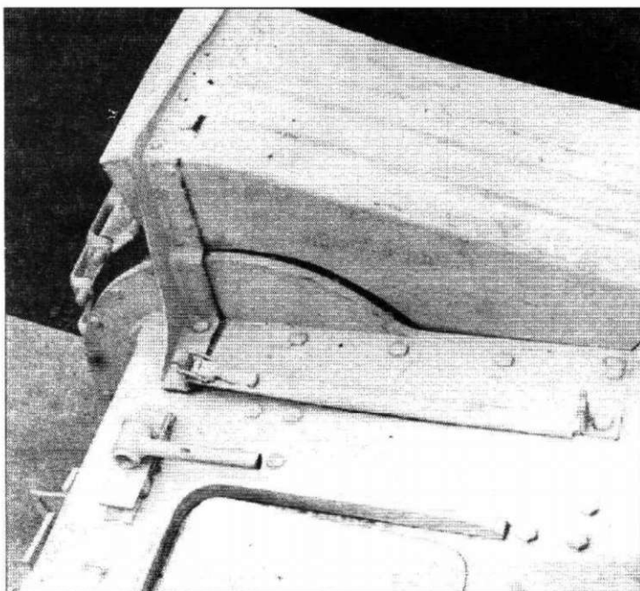
Крепление правого надгусеничного крыла.
