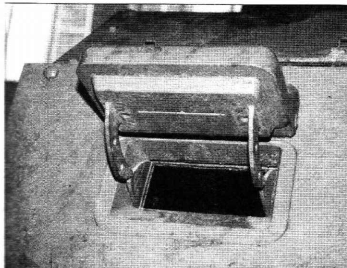
Открытый люк-пробка механика-водителя. За давностью лет исчезли механизм открывания люка и триплекс.
