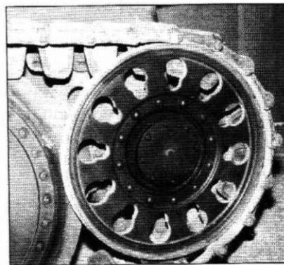
Ленивец танка Pz.Kpfw. 38(t) из музея в Лечанах, Чехия. Ленивцы истребителей танков «Мардер III» идентичны ленивцам танков Pz.Kpfw. 38(t).
