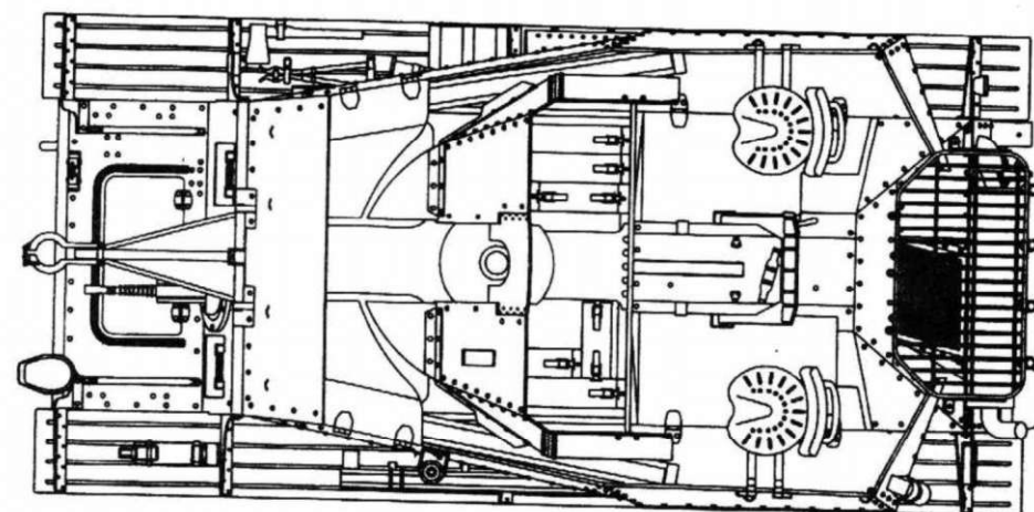
SdKfz 139 Panzerjager 38(t) für 7,62 cm Pak 36 Marder III
