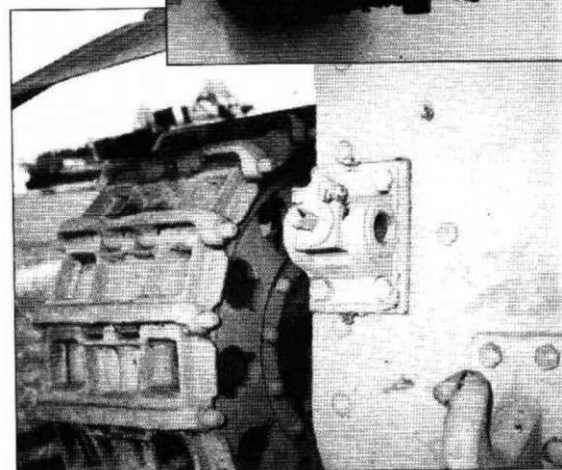
Механизм регулировки натяжения гусеницы. Хорошо видны траки. Отсутствует котак механизма регулировки натяжения. Абердин.
