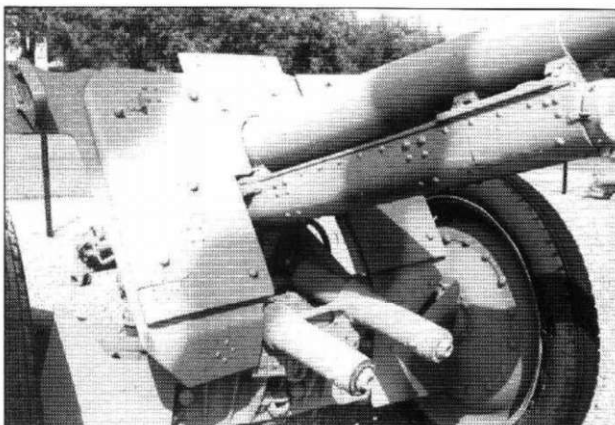
Орудийный щит противотанковой пушки 7,62 см Rak-36.
