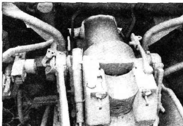
Вид сзади сверху на казенную часть орудия. Справа виден спусковой механизм с отверстием для крепления шнура. Сверху справа - рычаг затвора.
