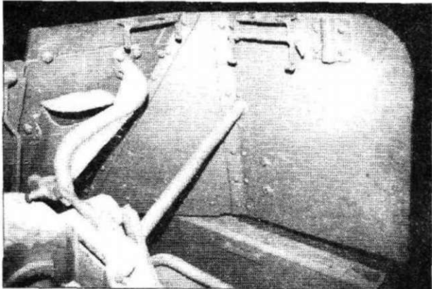
Правая внутренняя часть орудийного щита. В верхней части щита расположены кронштейны для перископических наблюдательных приборов и гнездо для дуги под теит. Самюр.
