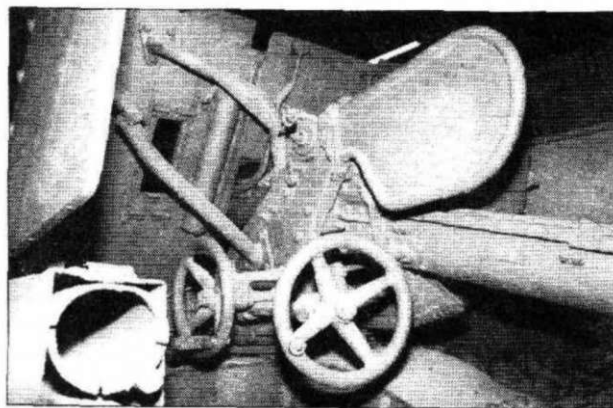
Еще один снимок левой части пушки, справа - штурвальчик горизонтального наведения, слева - штурвальчик вертикального наведения.
