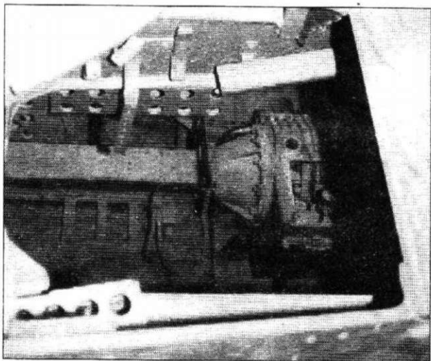
Интерьер отсека механика-водителя. Почти все оборудование на машине из Самюра отсутствует.
