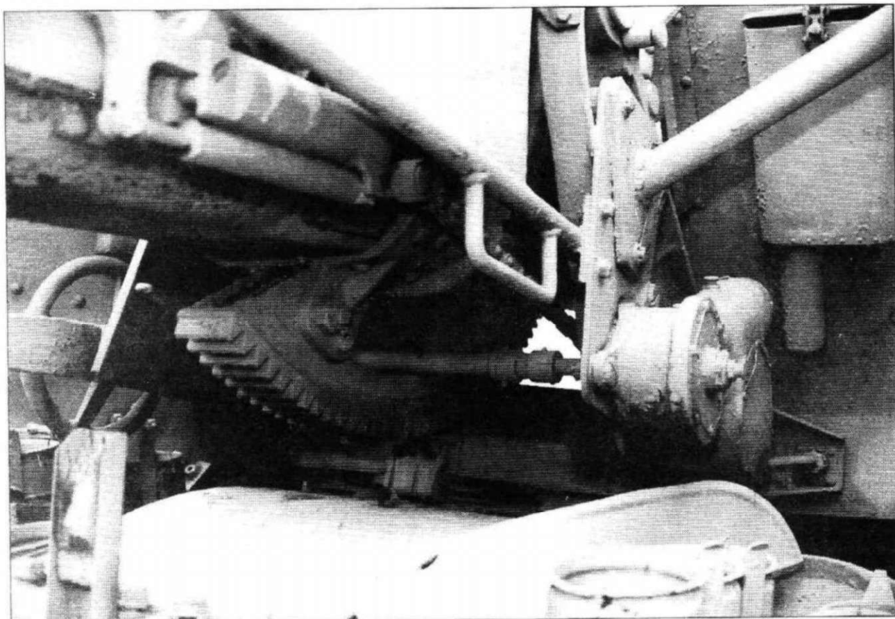
Крупный план механизма вертикального наведения. Абердин.
