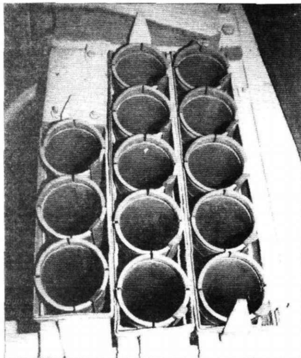
Правая основная боеукладка на 13 снарядов. Сямюр.
