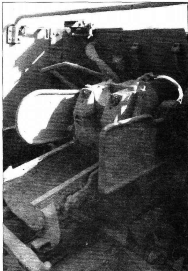
Казенная часть пушки, вид справа сзади.
