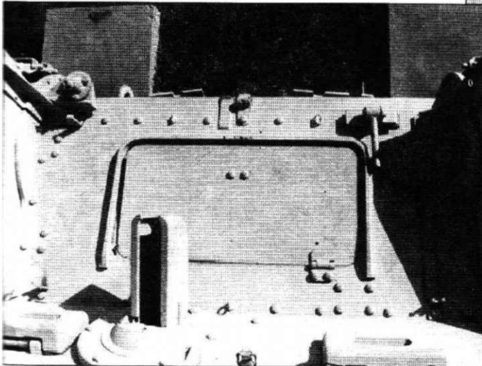
Лоб корпуса, вид сверху на люк доступа к тормозным устройствам.
