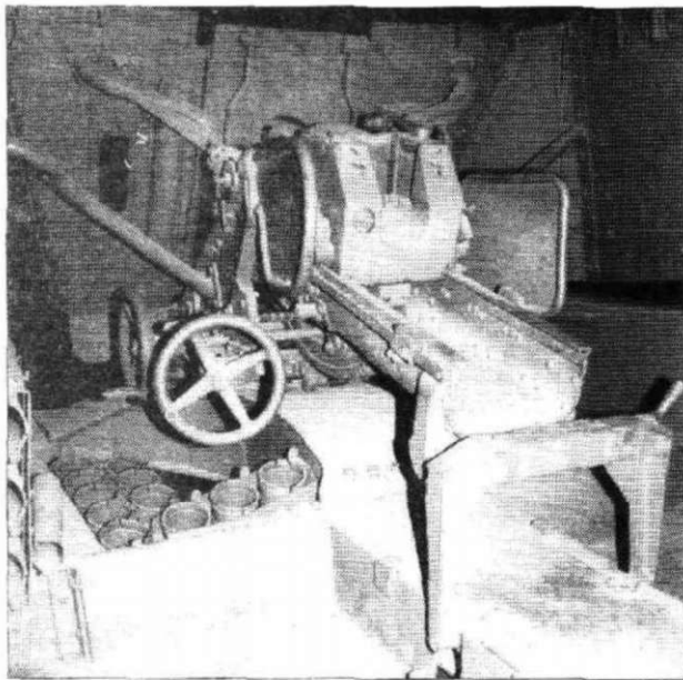
Вид слева на пушку и основную левую боеукладку на 11 снарядов. Обратите внимание на П-образный фиксатор казенной части пушки. Сямюр.
