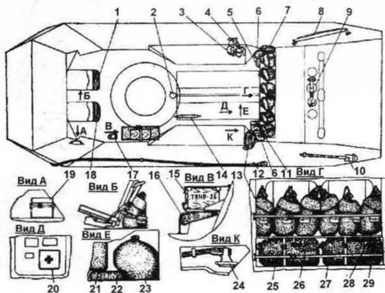
Укладка табельного имущества, шанцевого инструмента и ЗИП на БТР-70. Цифрами обозначены: 1. Мешок вещевой командира; 2. Бачок для питьевой воды; 3. и 13. Мешки вещевые десанта; 4. Огнетушитель углекислотный; 5. Ведро с воронкой и насосом для переливания бензина; 6. Бачок для масла; 7. Чехол с газожидкостным шлангом ДК-4Б; 8. Пила двуручная; 9. Блок лебедки; 10. Лопата; 11. Подставка домкрата большая; 12. Трос буксирный; 14. Шприц рычажно-плунжерный; 15. Ящик смотрового прибора ТНВО-2Б; 16. Прибор ДК-4КБ с принадлежностями комплекта в сумке; 17. Домкрат гидравлический; 18. Мешок вещевой водителя; 19. Сумка с противоголозом водителя; 20. Аптечка войсковая; 21. Чехол подвесной с инструментом и принадлежностями; 22. Чехол с инструментом и ЗИП малый; 23. Чехол с инструментом и ЗИП большой; 24. Топор; 25. Чехол для камеры колеса; 26. Камера колеса; 27. Мешок со спасательными жилетами; 28. Жилет спасательный; 29. Брезент подстилочный.
