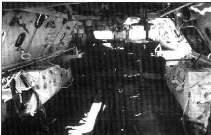
Вверху: Десантное отделение БТР-60ПБ. Вид в переднюю часть.
