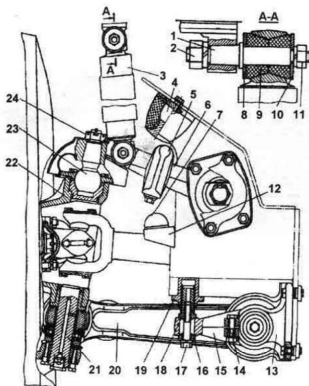
Подвеска первых и вторых (управляемых) колес на БТР-70. Цифрами обозначены: 1. Палец; 2, 11 и 24. Гайки; 3. Амортизатор; 4. Буфер сжатия; 5. Упор; 6. Верхний рычаг; 7. Буфер отдачи; 8 и 10. Шайбы; 9. Резиновая втулка; 12. Кронштейн буфера отдачи; 13. Кронштейн крепления нижнего рычага подвески; 14. Стяжной болт; 15. Муфта регулировочная; 16. Опорная шайба; 17. Болт стяжной; 18. Регулировочная втулка; 19. Пята; 20. Нижний рычаг; 21. Нижний шкворень поворотного кулака; 22. Поворотный кулак; 23. Верхний шкворень поворотного кулака.
