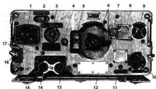
Передняя панель приемопередатчика Р-113.
