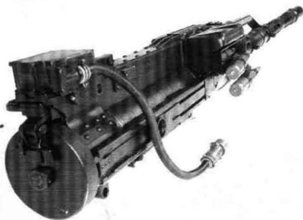
Общий вид пулемета КПВТ калибра 14,5-мм.
