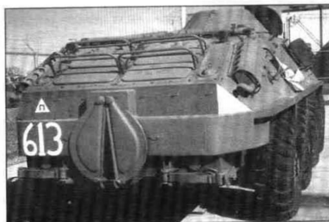
Кормовая часть румынского ТАВ-71М. Над жалюзи выхода охлаждающего воздуха установлено ограждение из изогнутого прута.
