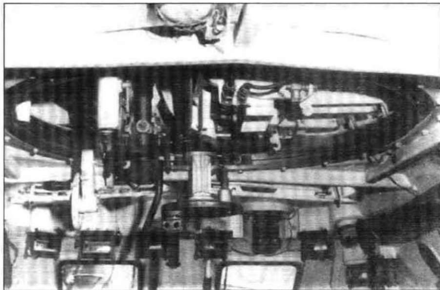
Вид на башиенную установку БТР-60ПБ изнутри.
