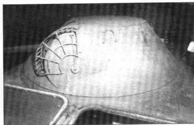
Кормовая часть румынского ТАВ-71М. Над жалюзи выхода охлаждающего воздуха установлено ограждение из изогнутого прута.
