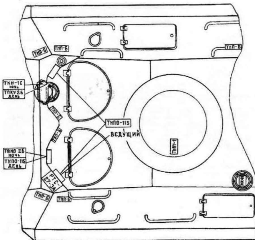
Схема расположения приборов наблюдения.
