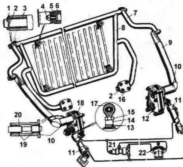
Волноотражательный щиток БТР-70. Цифрами обозначены: 1. Шплинт; 2. Шайба; 3. Втулка рычага; 4. Винт; 5. и 13. Регулировочные шайбы; 6. Буфер; 7. Ведомый рычаг; 8. Щиток; 9. Ведущий рычаг; 10. Опора; 11. Гидроцилиндр; 12. Редуктор правый; 14. Регулировочная втулка; 15. Контргайка; 16. Опора съемная; 17. Болт штока гидроцилиндров; 18. Редуктор левый; 19. Редуктор опоры; 20. Уплотнительное кольцо; 21. Гидрозамок; 22. Кран управления; 23. Ограничитель.
