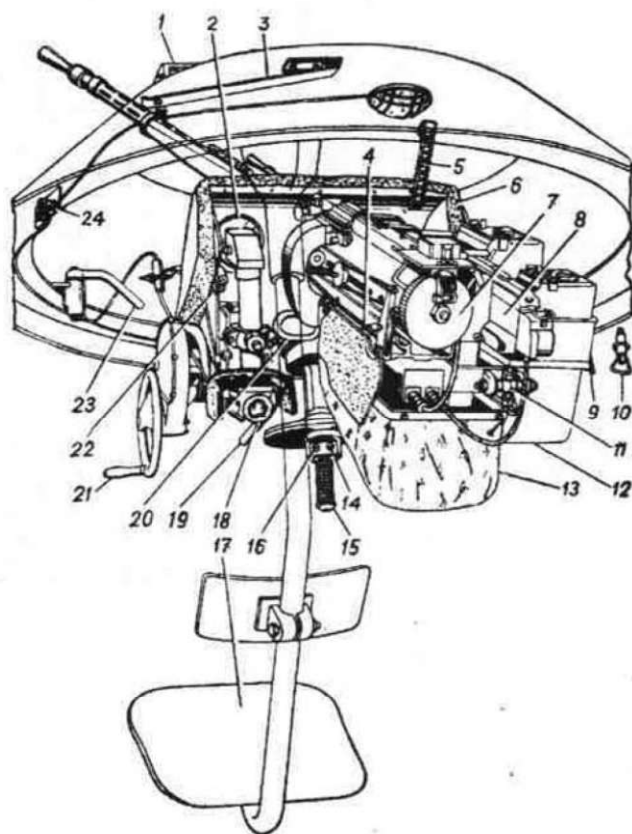
Общий вид башиенной установки. Цифрами обозначены: 1. Прибор наблюдения ТНПТ-1; 2. Обогреваемое защитное стекло прицела; 3. Планка стопора люльки по-походному; 4. Штифт; 5. Уравновешивающее устройство; 6. Уплотнение маски; 7. Пулемет КПВТ; 8. Пулемет ПКТ; 9. Защелка коробкодержателя; 10. Стопор башии по-походному; 11. Регулировочный механизм; 12. Патронная коробка; 13. Гильзозвеньесборник; 14. Кнопка электроспуска пулемета ПКТ; 15. Рукоятка маховика поворотного механизма; 16. Кнопка электроспуска пулемета КПВТ; 17. Сиденье стрелка; 18. Прицел; 19. Рукоятка тормоза подъемного механизма; 20. Рукоятка перезарядки; 21. Рукоятка маховика подъемного механизма; 22. Рукоятка стеклоочистителя; 23. Рукоятка тормоза погона; 24. Электрощиток башии.
