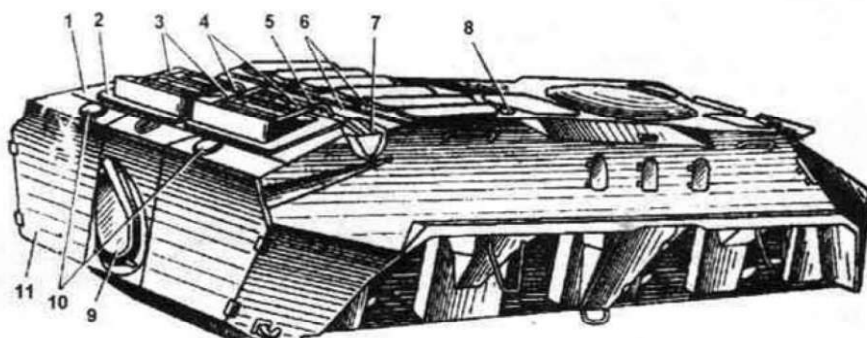
Корпус БТР-70 (вид сзади справа). Цифрами обозначены: 1. Задний съемный лист крыши; 2. Крышка жалюзи воздухоотвода; 3. Защитные решетки жалюзи; 4. Крышки лючков заливных горловин системы охлаждения; 5. Съемный надмоторный лист крыши; 6. Крышки надмоторных люков (с крышками воздухопритоков); 7. Съемная балка листов крыши отделения силовой установки; 8. Гнездо антенны; 9. Заслонка водомета; 10. Крышки заправочных горловин бензобаков; 11. Крышка отсека бензобака.
