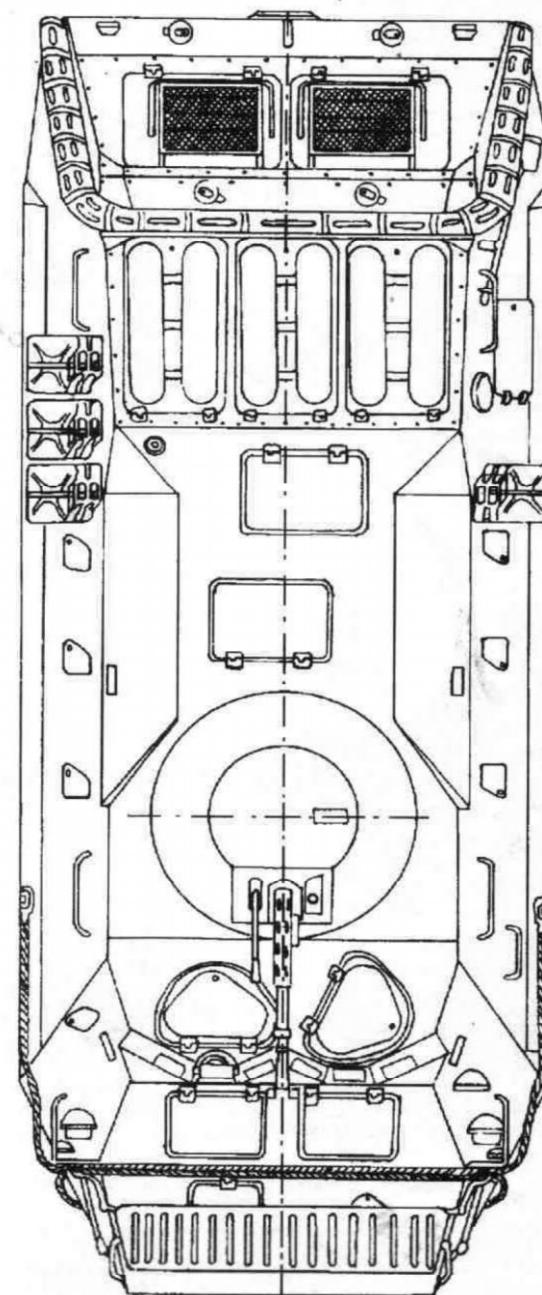
БТР-70 Масштаб 1:35
