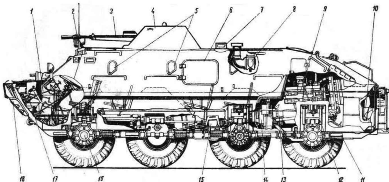
Схема общего устройства бронетранспортера БТР-60ПБ. Цифры обозначены: 1. Отделение управления; 2. Осветитель; 3. Крупнокалиберный пулемет; 4. Башенная установка; 5. Крышки лючков для стрельбы; 6. Крышка десантного люка; 7. Смотровой прибор десанта; 8. Фильтровентиляционная установка; 9. Двигатель; 10. Водомет; 11. Торсион подвески; 12. Амортизаторы; 13. Сцепление; 14. Коробка передач; 15. Раздаточная коробка; 16. Колесный редуктор и тормоз; 17. Лебедка; 18. Волноотражательный щит.
