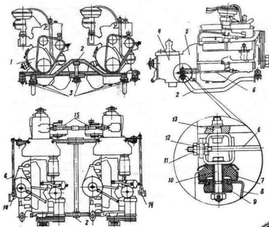
Силовая установка и ее крепление в бронетранспортере БТР-60ПБ. Цифрами обозначены: 1. Двигатель; 2. Промоторная рама; 3. Опоры рамы с резиновыми подушками; 4. Коробка передач; 5. Сцепление; 6. Тяга, соединяющая раму с корпусом БТР; 7. Верхняя резиновая подушка; 8. Кронштейн корпуса для крепления рамы; 9. Нижняя резиновая подушка; 10. Болт крепления рамы; 11. Гайка тяги; 12. Контргайка тяги; 13. Болт крепления двигателя к раме; 14. Боковые кронштейны корпуса; 15. Коробки отбора мощности на привод водомета.
