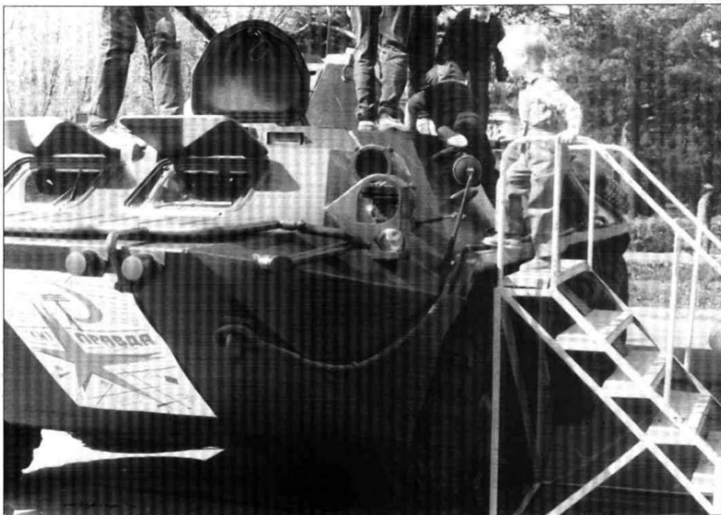
Башня БТР-70 была унифицирована с БРДМ-2 и БТР-60. Все фото - Андрея Аксенова.
