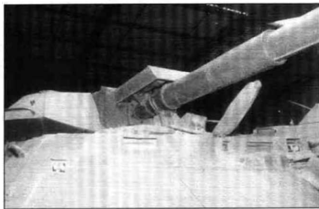
На фото хорошо видны тормозные устройства пушки прикрытые сверху броневой коробкой.
