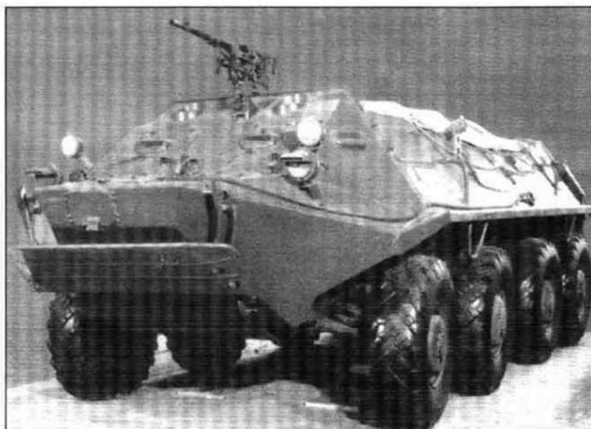
Опытный образец БТР-60П в экспозиции танкового музея в Кубинке.
