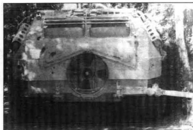
Корма БТР-60, заслонки водомета подняты. Обратите внимание на откинутое буксирное устройство (справа).
