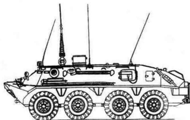
Схема общего вида машины управления БТР-60ПУ12.
