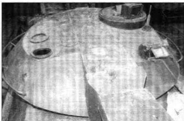
Вид на башню сверху. В ее правой части размещались командир и наводчик. На переднем плане виден прицел 1ПН22 (как на БМП-1), за ним командирская башенка и основание антенны. Хорошо видно, что передняя часть башни плоская и имеет большой угол наклона.
