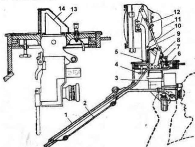
Осветитель ОУ-3ГА-2 прибора наблюдения командира. Цифрами обозначены: 1. Кронштейн; 2. Корпус осветителя; 3. Кронштейн крепления осветителя с прибором; 4. Продольные прорезы цапфы.
