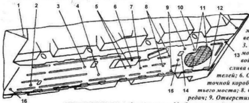
Днище БТР-70. Цифрами обозначены: 1. Отверстие для слива охлаждающей жидкости из переднего отопителя; 2. Отверстие для слива масла из первого моста; 3. Отверстие для слива масла из второго моста; 4. Отверстие для слива масла из правой раздаточной коробки; 5. Отверстия для слива охлаждающей жидкости из задних отопителей; 6. Отверстие для слива масла из левой раздаточной коробки; 7. Отверстие для слива масла из третьего моста; 8. Отверстия для слива масла из коробок передач; 9. Отверстия для слива масла из двигателей и выпуска газов из пускового подогревателя; 10. Отверстие для слива масла из четвертого моста; 11. Отверстие для слива охлаждающей жидкости из теплообменников; 12. Отверстия для слива топлива из баков; 13. Отверстие для слива воды из корпуса; 14. Лючок для доступа к гайкам крепления карданного вала привода четвертого моста, к шлангу и крану котла пускового подогревателя; 15. Отверстие для слива воды из котла пускового подогревателя; 16. Отверстие для слива воды из корпуса. Отверстия 2, 3, 4, 6, 7, 8, 9, 10, 12, 13 и 15 закрываются резьбовыми пробками.
