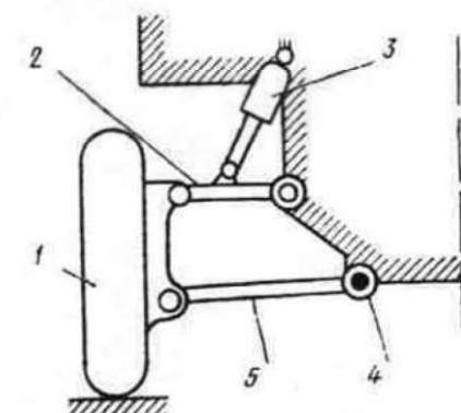
Схема независимой двухрычажной подвески бронетранспортера. Цифрами обозначены: 1. Колесо и картер колесного редуктора; 2. Верхний рычаг подвески; 3. Амортизатор; 4. Тorsiон; 5. Нижний рычаг подвески.
