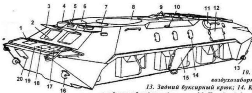
Корпус БТР-70 (вид спереди слева). Цифрами обозначены: 1. Крышка люка лебедки; 2. Ветровое стекло смотрового люка; 3. Крышка смотрового люка; 4. Гнездо прибора наблюдения командира; 5. Гнездо прибора наблюдения ТНПО-115; 6. Крышка люка командира; 7. Крышка люка водителя; 8. Люк башенной установки; 9. Крышки верхних люков десанта; 10. Крышки люков для стрельбы; 11. Колпак воздухозаборника ФВУ; 12. Крышка люка фильтра ФВУ; 13. Задний буксирный крюк; 14. Крышка бокового люка десанта; 15. Гнездо прибора наблюдения десанта; 16. Передний буксирный крюк; 17. Крышка люка главных цилиндров сцепления; 18. Крышка люка главных цилиндров рабочей тормозной системы; 19. Волноотражательный щиток; 20. Крышка люка выдачи троса лебедки.
