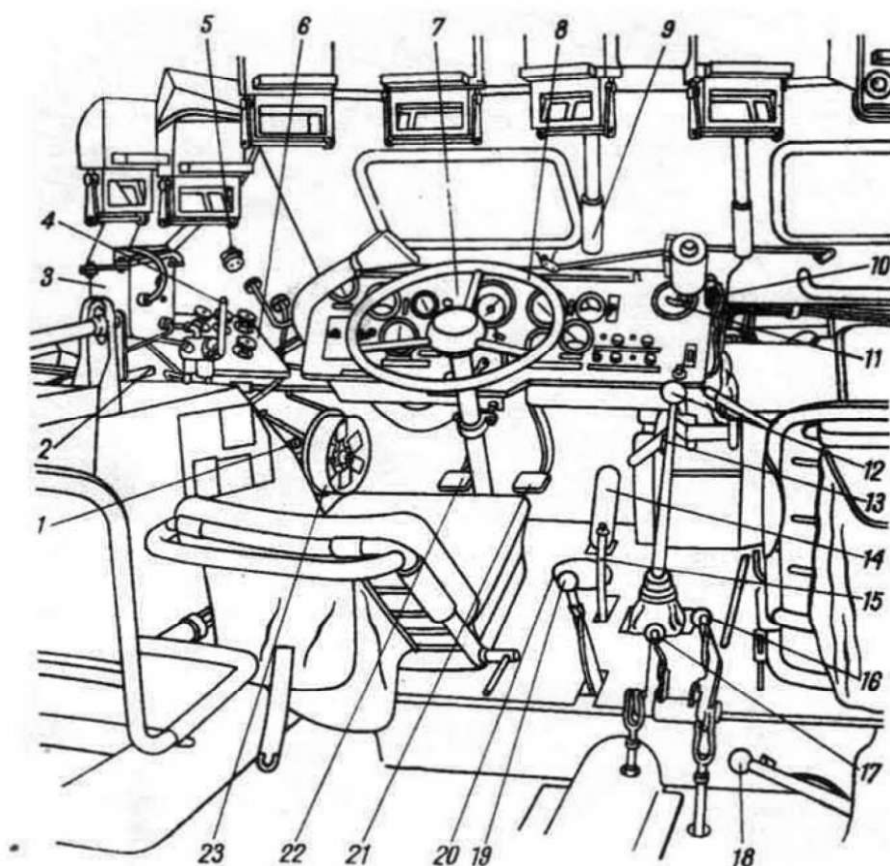
Отделение управления БТР-60ПБ. Цифрами обозначены: 1. Кнопка управления воздушной заслонкой карбюратора; 2. Рукоятка управления жалюзи; 3. Блок питания прибора ночного видения водителя; 4. Рукоятка крана управления заслонками водомета; 5. Розетка переносной лампы; 6. Блок шинных кранов; 7. Щиток приборов; 8. Рулевое колесо; 9. Рукоятка крышки смотрового люка водителя; 10. Включатель стеклоочистителя; 11. Рычаг ручного привода стеклоочистителя; 12. Рычаг переключения передач; 13. Рычаг привода волноотражателя; 14. Педаль управления дроссельными заслонками карбюратора; 15. Рычаг стояночного тормоза; 16. Рычаг включения передних мостов; 17. Рычаг переключения передач в раздаточных коробках; 18. рычаг управления лебедкой; 19. Рычаг управления водометом; 20. Люк для слива конденсата из воздушного баллона; 21. Педаль рабочего тормоза; 22. Педаль сцепления; 23. Передний отопитель.
