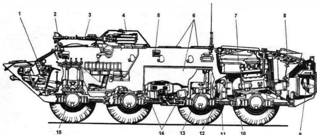
Схема общего устройства бронетранспортера БТР-70. Цифры обозначены: 1. Отделение управления; 2. Осветитель; 3. Крупнокалиберный пулемет; 4. Башенная установка; 5. Смотровый прибор; 6. Крышки десантных люков; 7. Двигатель; 8. Радиатор и вентилятор; 9. Водомет; 10. Сцепление; 11. Коробка передач; 12. Торсион подвески; 13. Амортизатор; 14. Раздаточная коробка; 15. Колесный редуктор.
