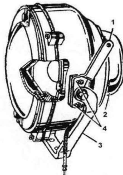
Осветитель ОУ-3ГА-2 прибора наблюдения командира. Цифрами обозначены: 1. Кронштейн; 2. Корпус осветителя; 3. Кронштейн крепления осветителя с прибором; 4. Продольные прорезы цапфы.
