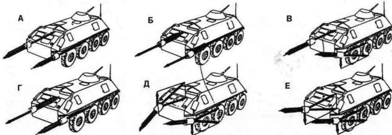
Режимы работы забортных водометов опытного БТР-60ПБ.
