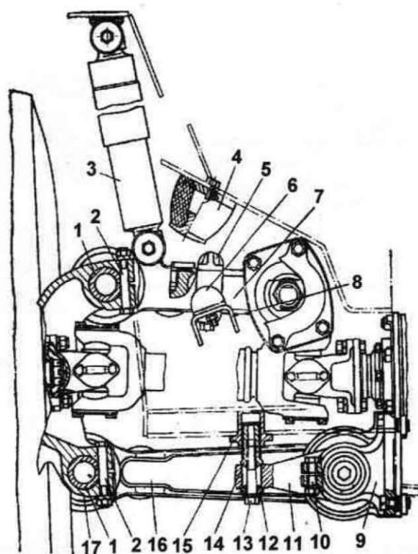
Подвеска третьих и четвертых колес на БТР-70. Цифрами обозначены: 1. Соединительная ось; 2. Стяжные болты; 3. Амортизатор; 4. Буфер сжатия; 5. Упор; 6. Буфер отдачи; 7. Верхний рычаг; 8. Кронштейн буфера отдачи; 9. Кронштейн крепления нижнего рычага; 10. Стяжной болт; 11. Регулировочная муфта; 12. Опорная шайба; 13. Стяжной болт; 14. Регулировочная втулка; 15. Пята; 16. Рычаг нижний; 17. Корпус редуктора.
