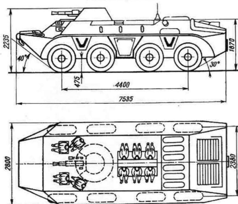
Основные размеры бронетранспортера БТР-70 и схема размещения в нем боевого расчета.
