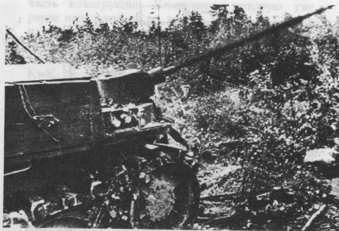
Метание зажигательной смеси из PzKpfw II (F) "Фламинго". Жидкость еще не подожжена, так как для эффективного ее применения необходимо было сначала залить ею цель, а уже потом - поджечь.
